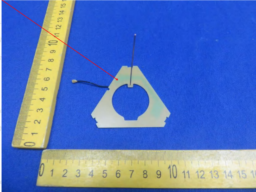
Lora ANT
