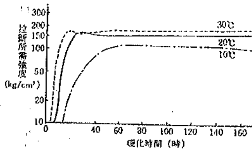
圖 II 2.3 常溫時の硬化特性 硬化劑混合率 100phr
