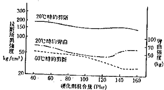
圖 II 2.1 硬化劑混合量と粘着力強度 (在20°C七天的硬化) 試験片: 軟鋼板 (25×100×1.6mm) (Over-lap)12.5mm
