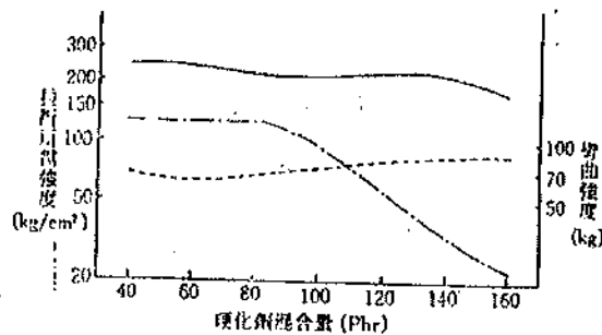
圖 II 2.2 硬化劑混合量と粘着力強度 (在80°C一小時的硬化) 試験片: 以及其他同圖 II 2.1
