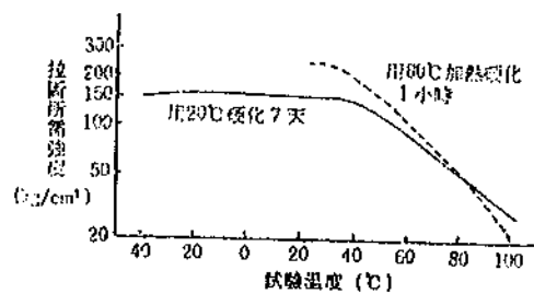
圖 II 2.5 耐熱特性 硬化劑混合率 100phr
