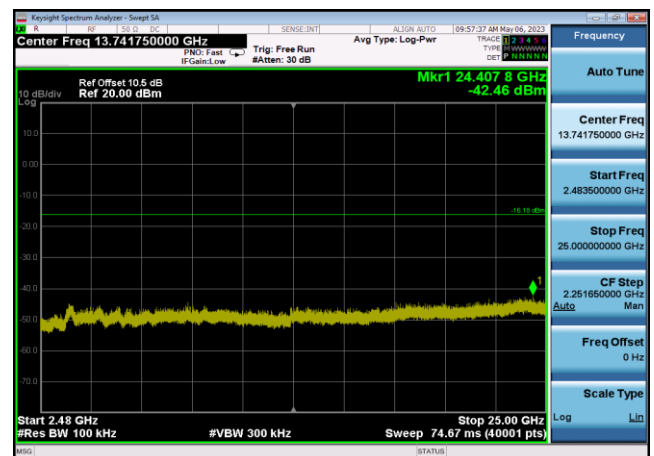
,Plot 4,2483.5MHz~25000MHz-802.11n(HT20),2462MHz,Ant0
