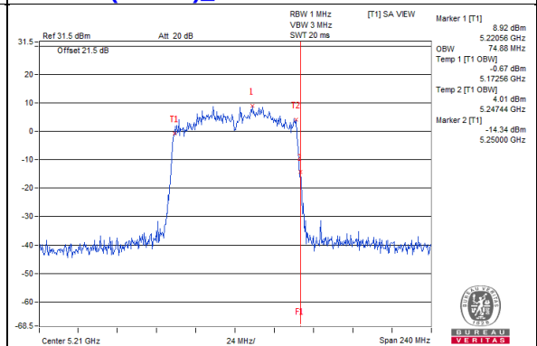
802.11ac(VHT80)_Chain3 / CH42
