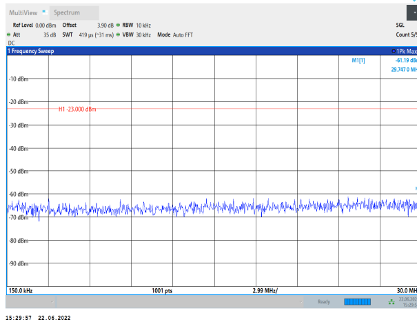
Band12-10MHz-QPSK-23060-1RB#0-Range2:0.15~30MHz
