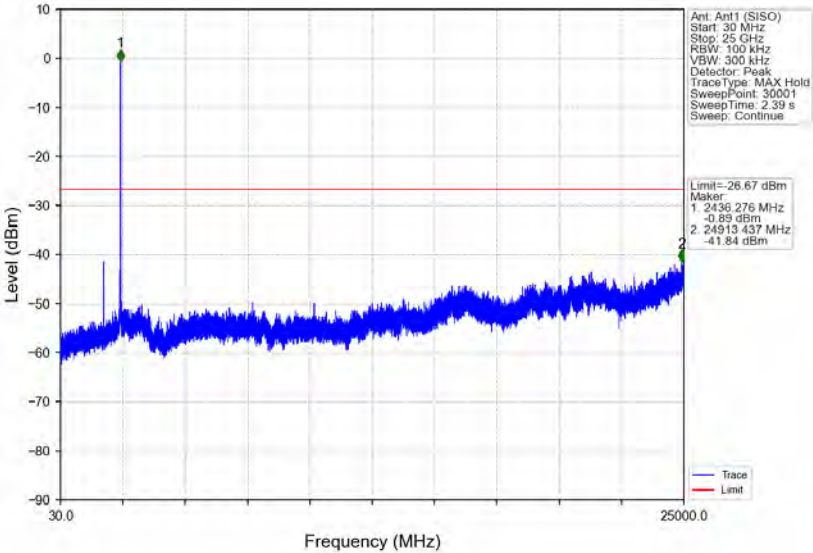
802.11g_MCH_2437MHz_Ant1 (SISO)_NTNV
