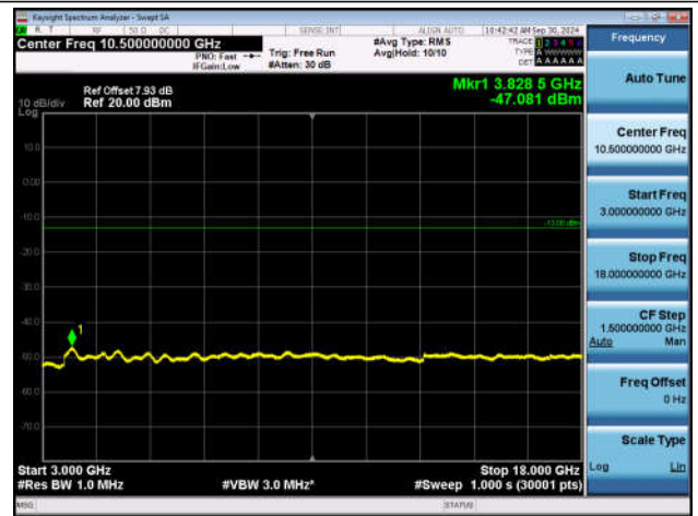
EGPRS1900-512-2-3000~18000MHz-PASS
