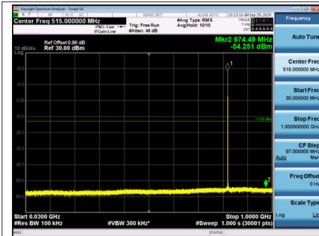
GSM850-128-5-30~1000MHz-PASS
