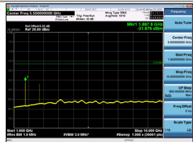
GSM850-251-5-1000~10000MHz-PASS
