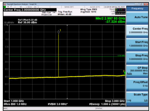
GSM1900-512-0-1000~3000MHz-PASS
