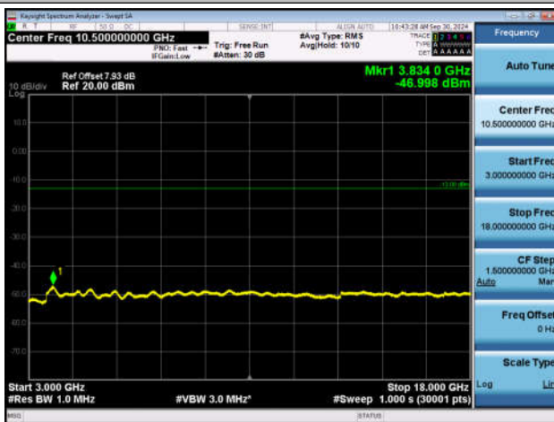
EGPRS1900-661-2-3000~18000MHz-PASS
