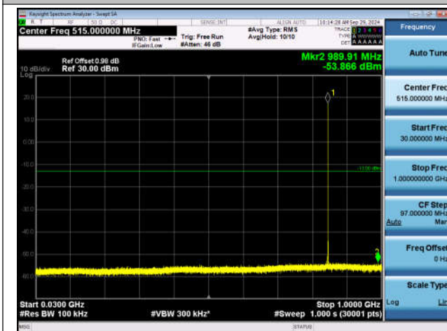
GSM850-251-5-30~1000MHz-PASS
