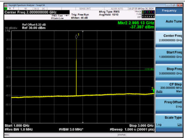
GSM1900-810-0-1000~3000MHz-PASS
