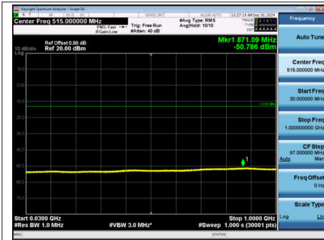
GSM1900-810-0-30~1000MHz-PASS
