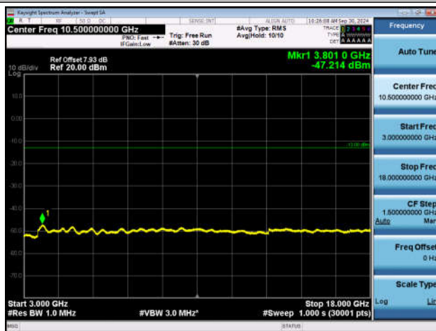
GSM1900-512-0-3000~18000MHz-PASS
