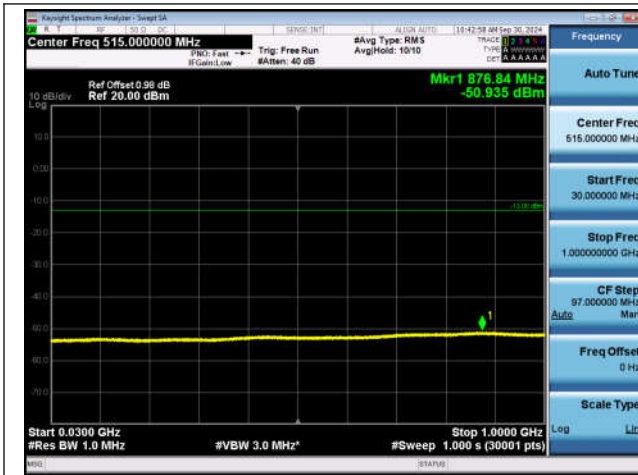
EGPRS1900-661-2-30~1000MHz-PASS
