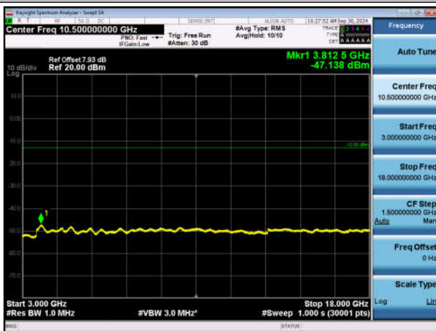
GSM1900-810-0-3000~18000MHz-PASS
