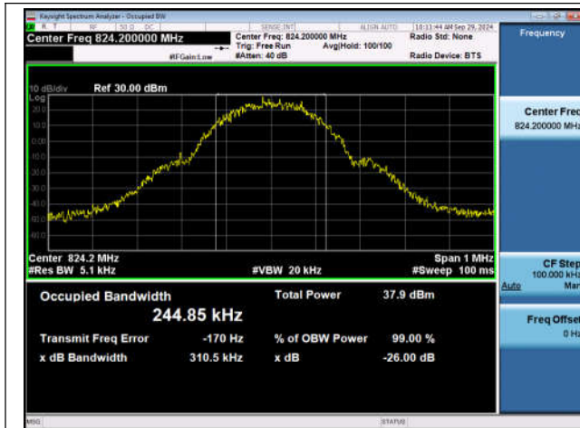
GSM850-128-5-PASS
