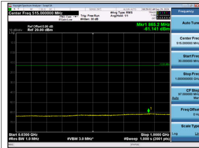
Band4-1312-30~1000MHz-PASS
