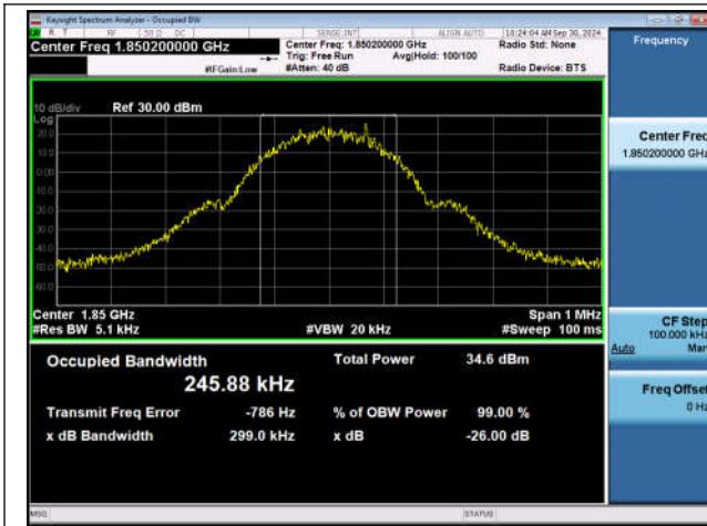
GSM1900-512-0-PASS
