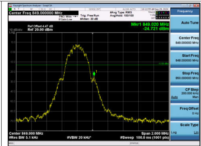
GSM850-251-5-PASS
