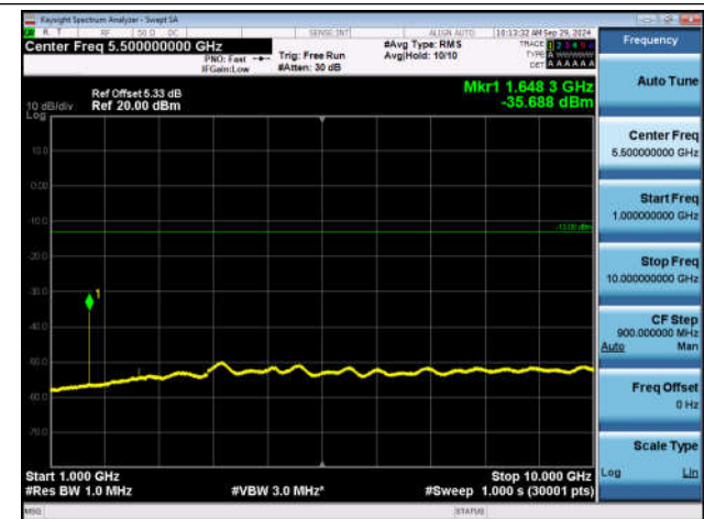
GSM850-128-5-1000~10000MHz-PASS
