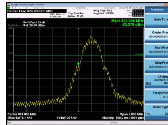
GSM850-128-5-PASS
