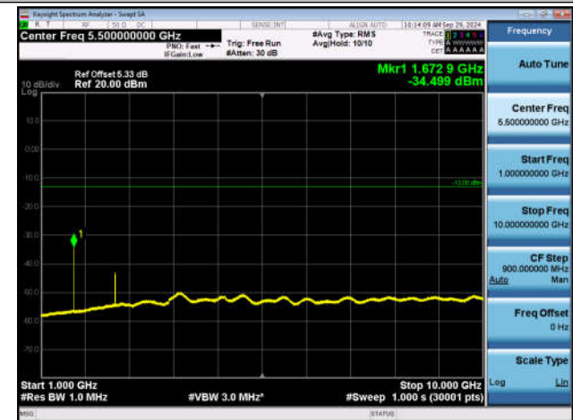
GSM850-190-5-1000~10000MHz-PASS
