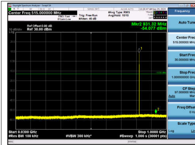
EGPRS850-128-8-30~1000MHz-PASS
