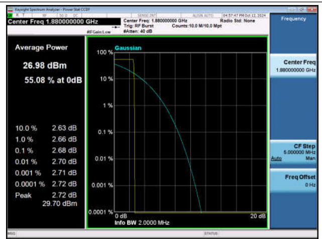
GSM1900-661-0-PASS
