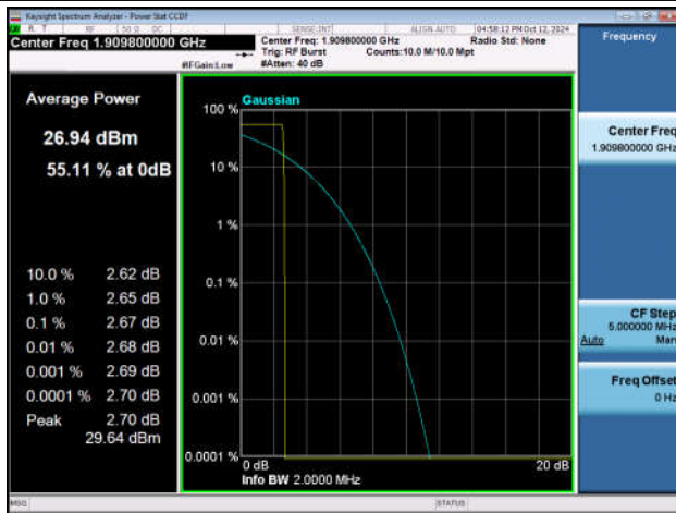
GSM1900-810-0-PASS
