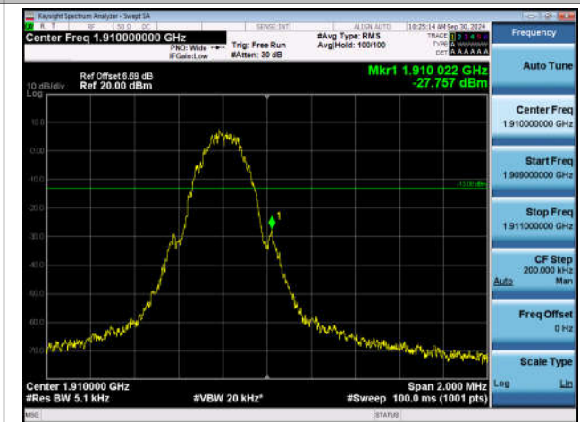
GSM1900-810-0-PASS
