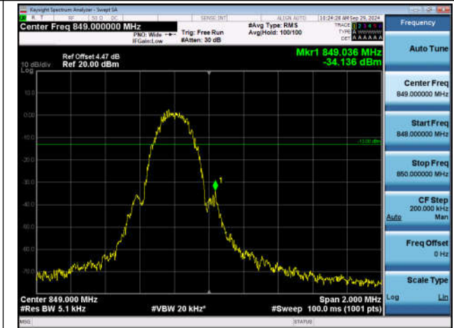
EGPRS850-251-8-PASS
