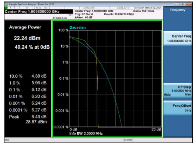
EGPRS1900-810-2-PASS
