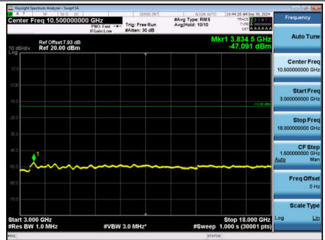
EGPRS1900-810-2-3000~18000MHz-PASS
