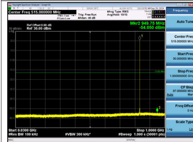
GSM850-190-5-30~1000MHz-PASS
