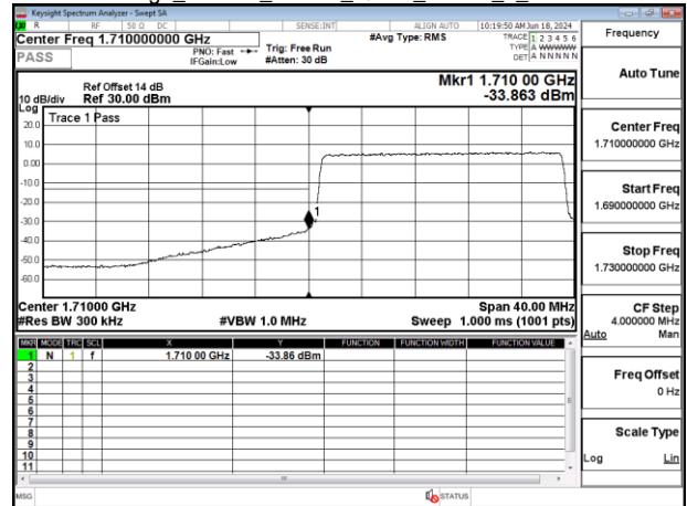
Band Edge_Band66_20MHz_QPSK_RB100_0_CH132572
