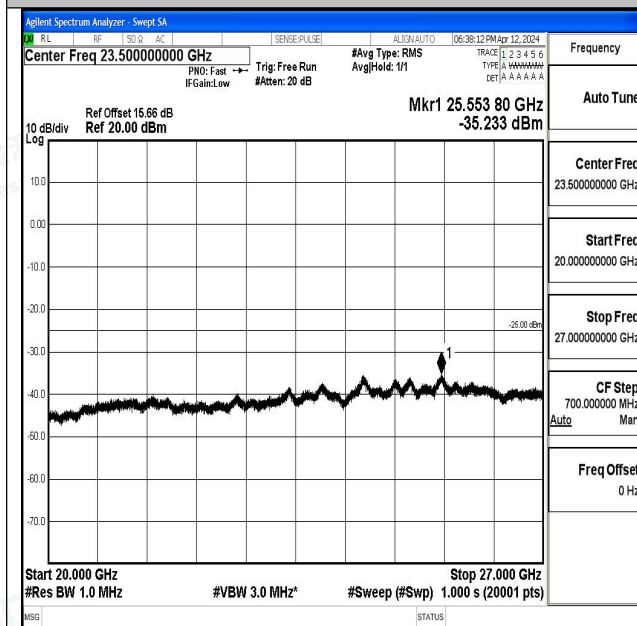
Band7_20MHz_QPSK_20850_1RB#0_20000~27000_20 000~27000
