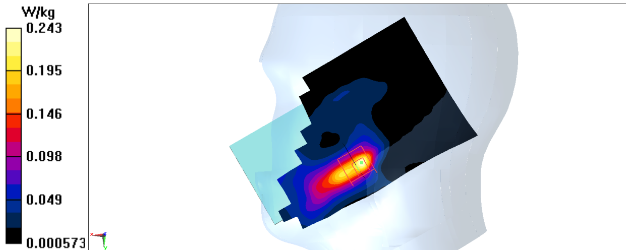
Fig.9 LTE Band7
