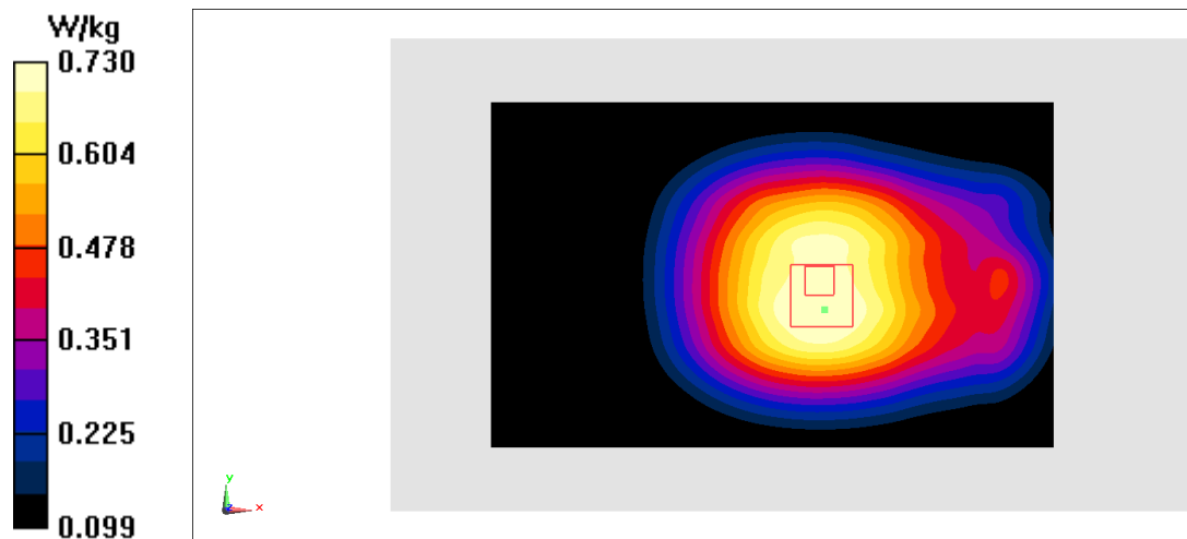
Fig.6 WCDMA 850
