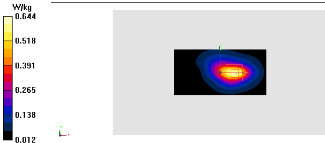
Fig.8 WCDMA1900
