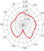
2450.000MHz E1
