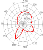
2450.000MHz E2
