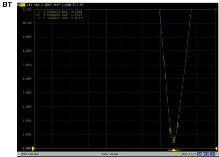
VSWR
