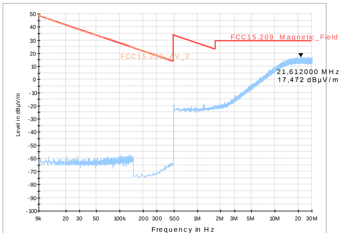
FCC15.209_magn hor+vert
