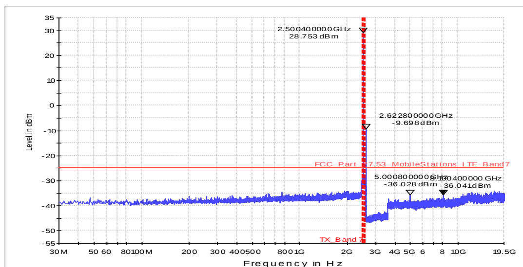
Fula2_FCC_27_LTE_Bd7_Scan2_30MHz_19.5GHz
