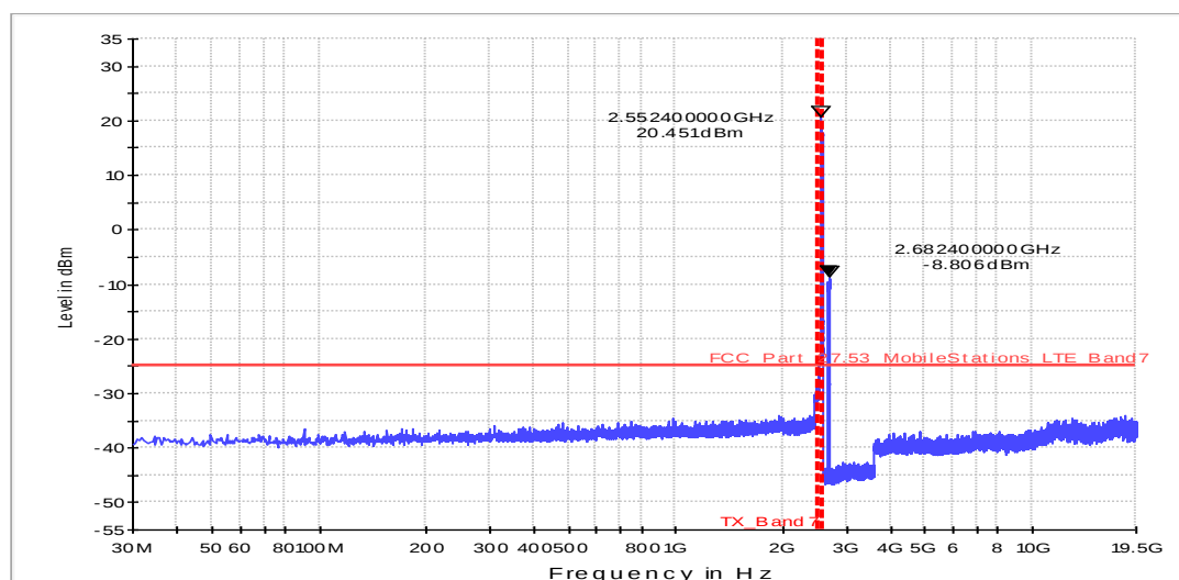
Fula2_FCC_27_LTE_Bd7_Scan2_30MHz_19.5GHz
