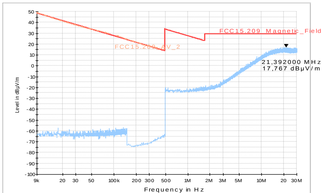
FCC15.209_magn hor+vert
