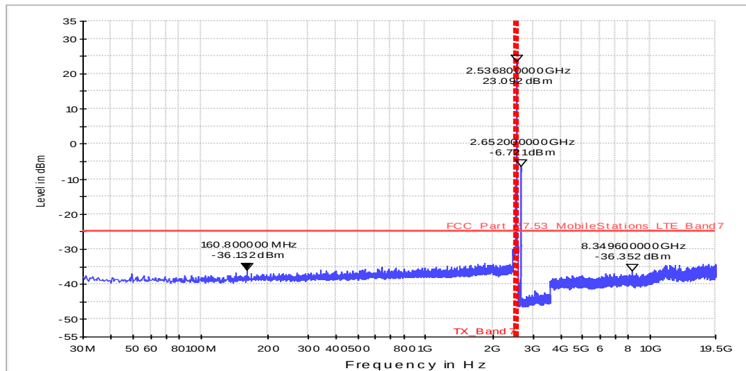
Fula2_FCC_27_LTE_Bd7_Scan2_30MHz_19.5GHz
