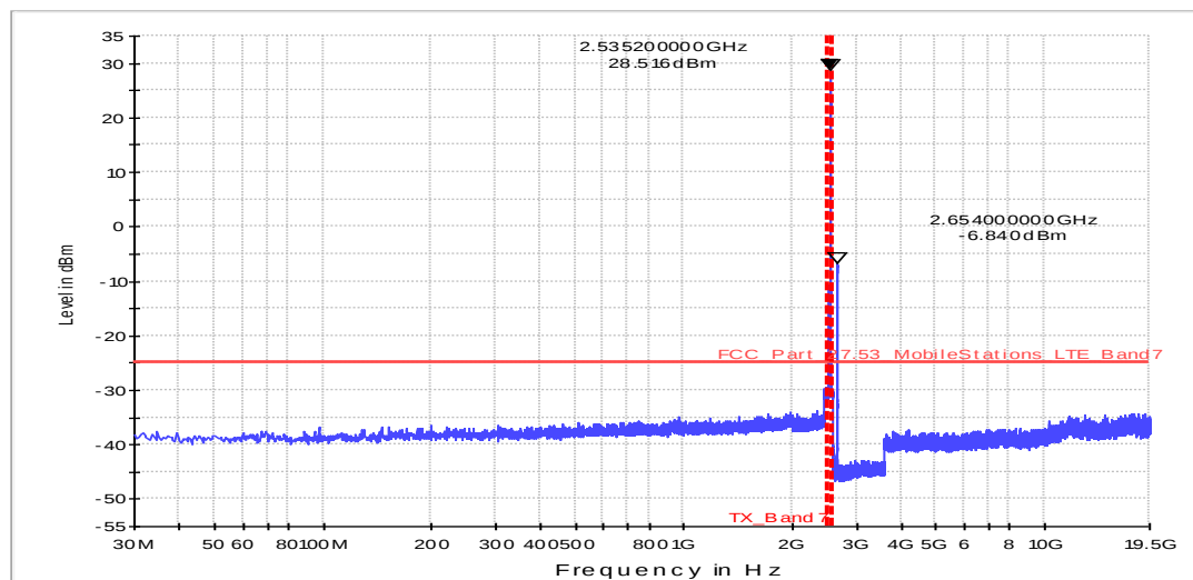
Fula2_FCC_27_LTE_Bd7_Scan2_30MHz_19.5GHz
