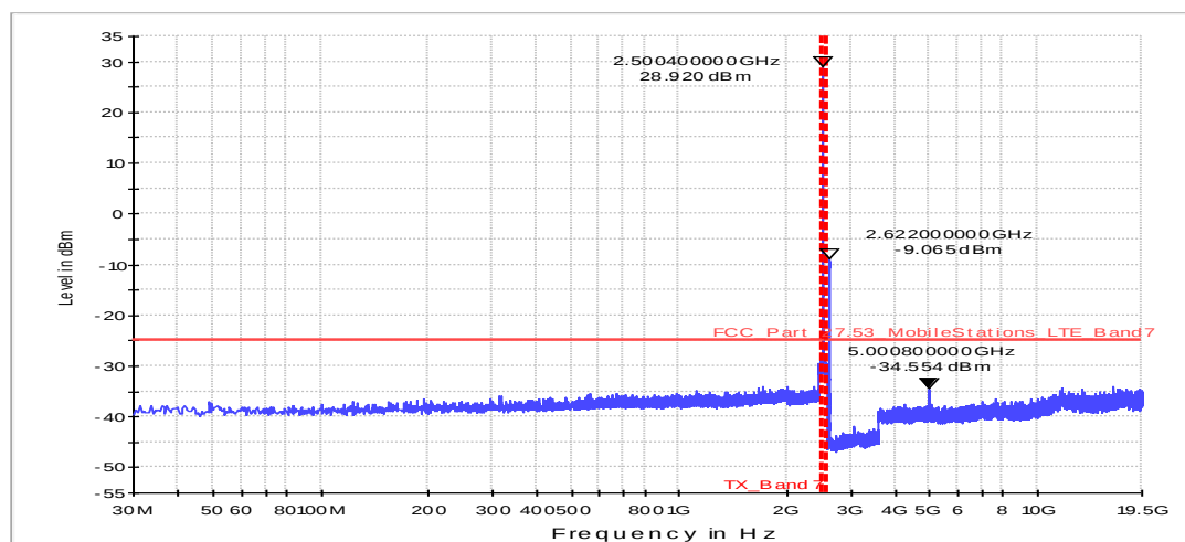
Fula2_FCC_27_LTE_Bd7_Scan2_30MHz_19.5GHz
