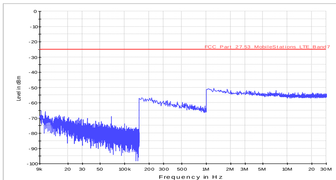
Fula2_FCC_27_LTE_Bd7_Scan1_9kHz_30MHz
