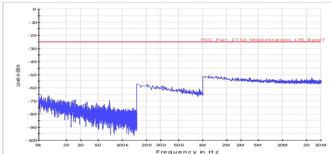
Fula2_FCC_27_LTE_Bd7_Scan1_9kHz_30MHz
