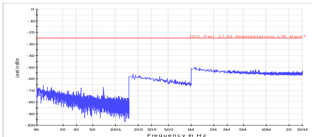
Fula2_FCC_27_LTE_Bd7_Scan1_9kHz_30MHz
