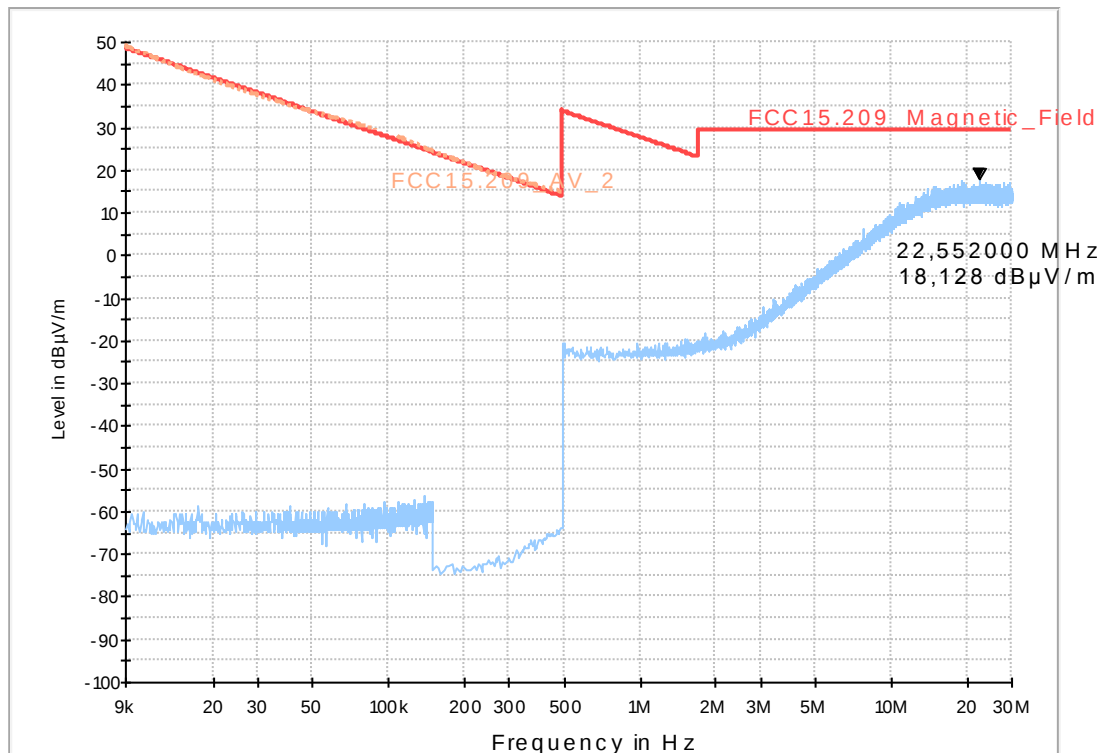
FCC15.209_magn hor+vert
