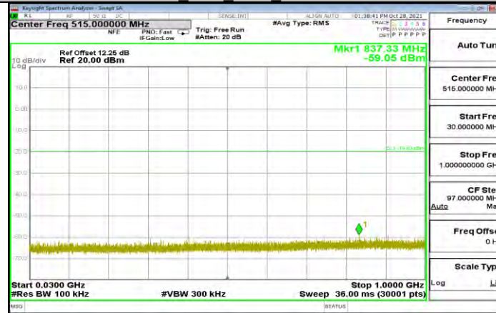
3DH5 Ant1 2441 30~1000
