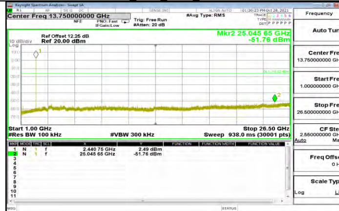
DH5 Ant1 2441 1000~26500
