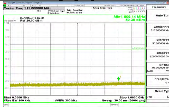
DH5 Ant1 2441 30~1000
