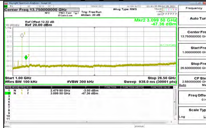
3DH5 Ant1 2480 1000~26500
