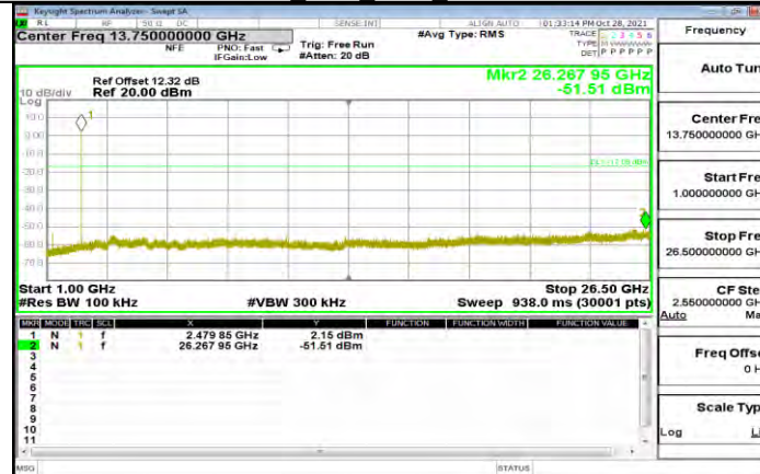
DH5 Ant1 2480 1000~26500
