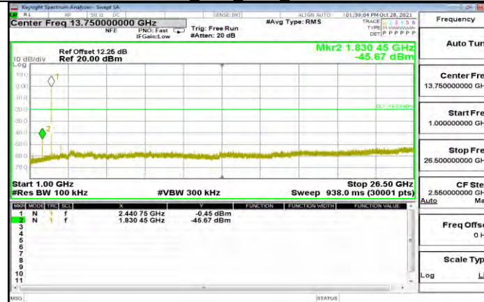
3DH5 Ant1 2441 1000~26500
