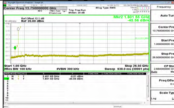
3DH5 Ant1 2402 1000~26500
