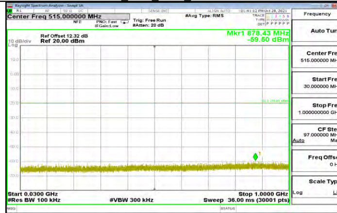
3DH5 Ant1 2480 30~1000
