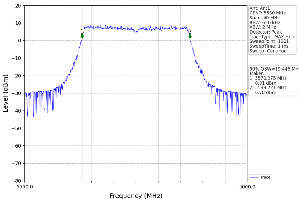
802.11be(EHT20)_MCH_5580MHz_RU242_Left_Ant1_NTNV
