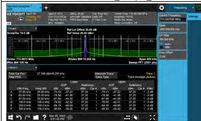
3dB Above AGC_ Output_4
