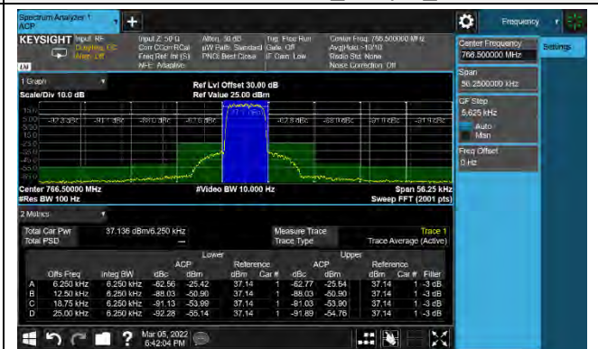
3dB Above AGC_ Output_3
