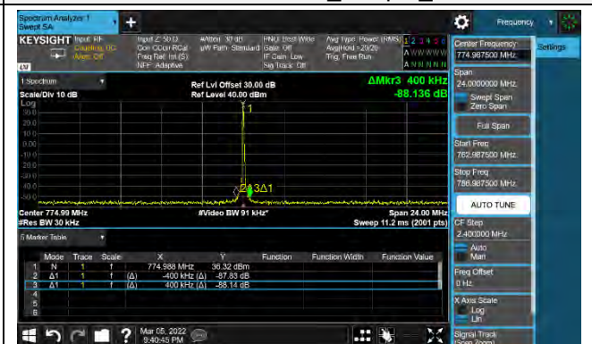
3dB Above AGC_ Output_3
