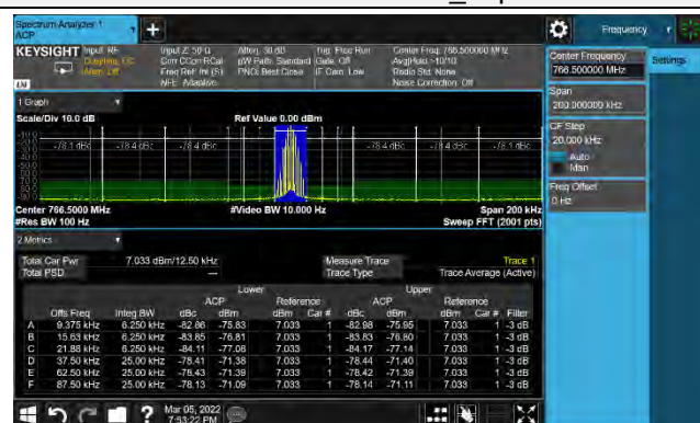
3dB Above AGC_ Output_2
