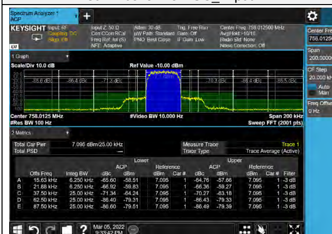
3dB Above AGC_ Output_2
