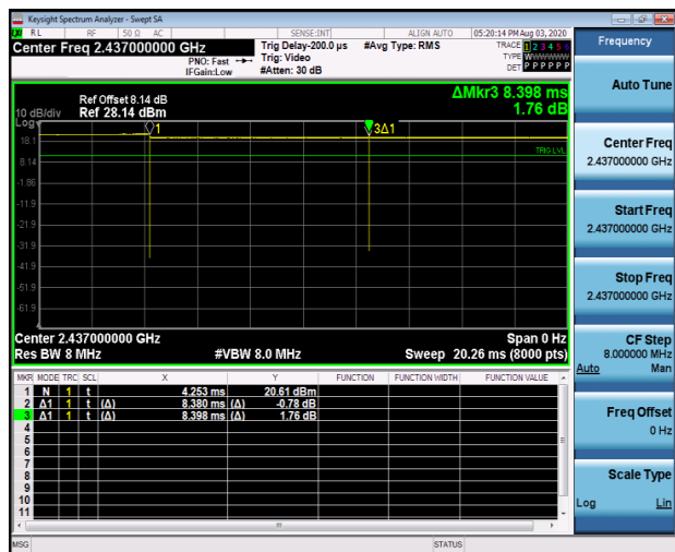
802.11b
