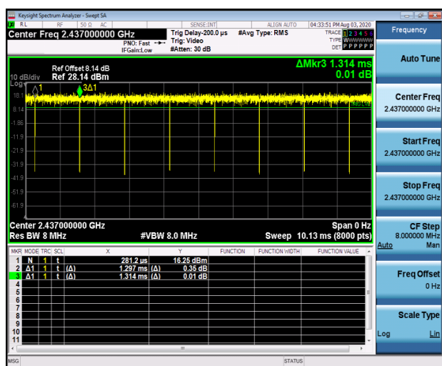
802.11n HT20
