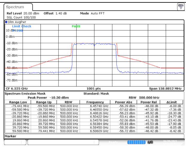
802.11ax (40MHz) 6525MHz Chain B NSS-4
