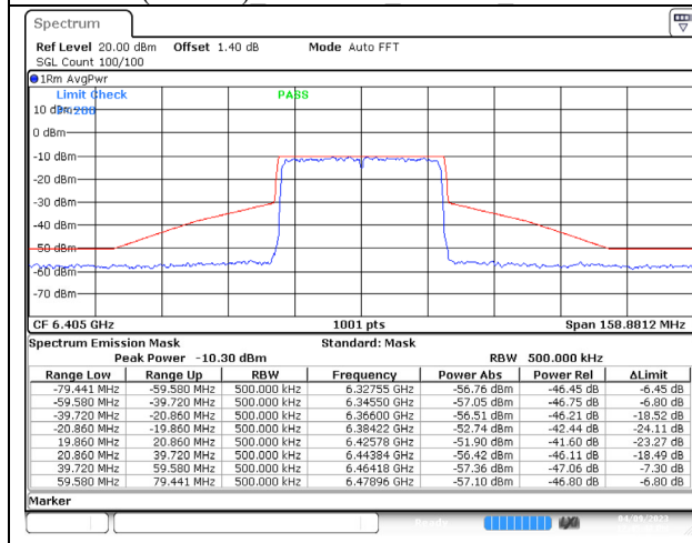
802.11ax (40MHz) 6405MHz Chain C NSS-4
