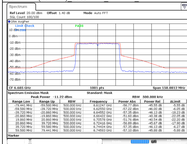
802.11ax (40MHz) 6685MHz Chain C NSS-4
