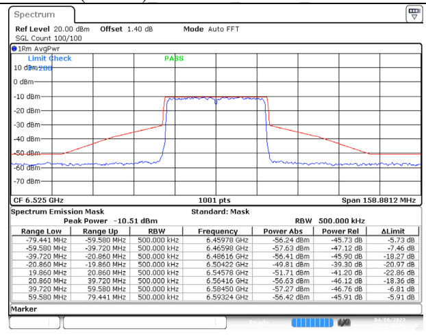
802.11ax (40MHz) 6525MHz Chain D NSS-4
