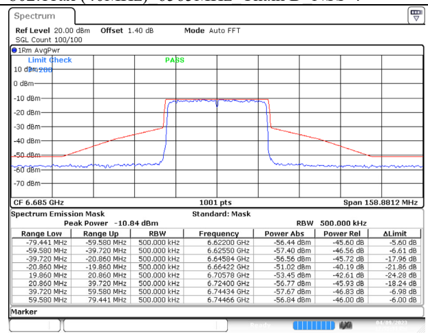
802.11ax (40MHz) 6685MHz Chain B NSS-4
