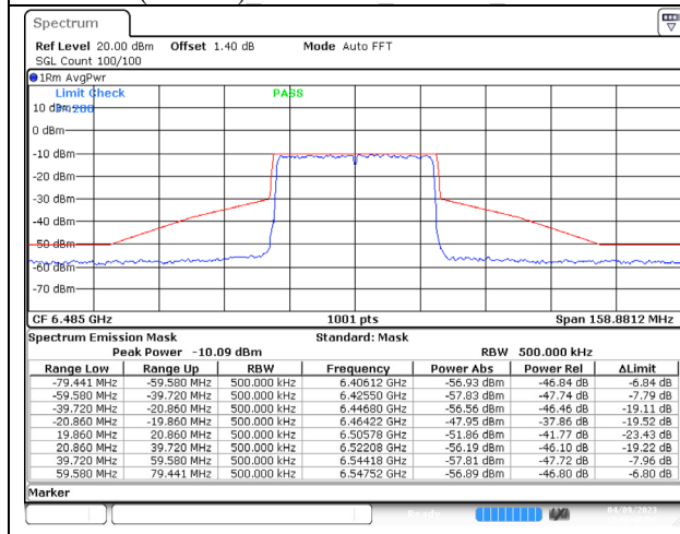
802.11ax (40MHz) 6485MHz Chain A NSS-4
