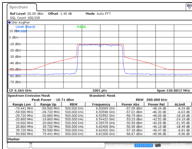
802.11ax (40MHz) 6565MHz Chain C NSS-4
