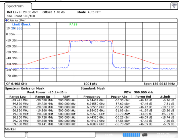
802.11ax (40MHz) 6405MHz Chain D NSS-4
