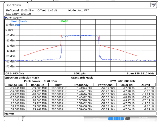
802.11ax (40MHz) 6485MHz Chain D NSS-4
