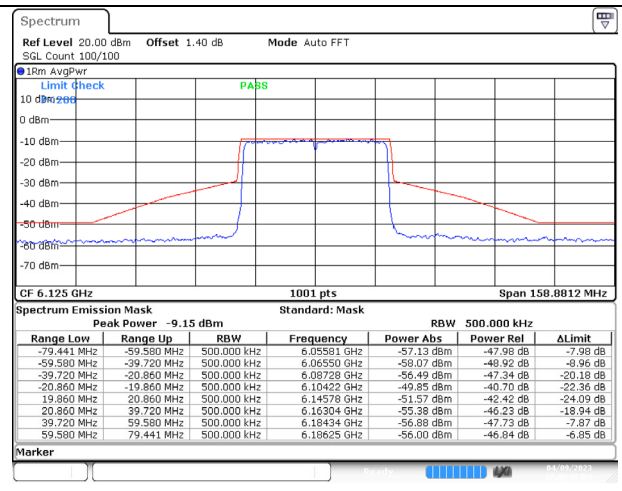
802.11ax (40MHz) 6125MHz Chain D NSS-4
