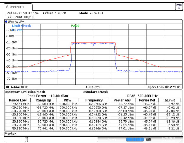
802.11ax (40MHz) 6565MHz Chain D NSS-4
