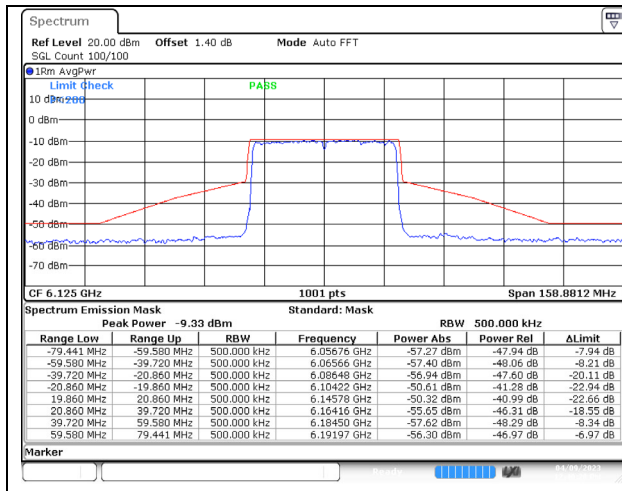
802.11ax (40MHz) 6125MHz Chain C NSS-4
