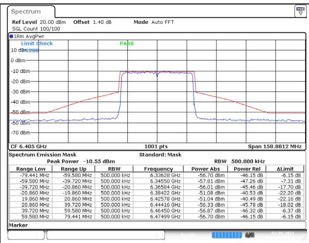
802.11ax (40MHz) 6405MHz Chain B NSS-4
