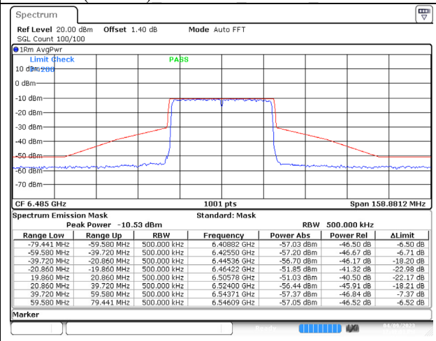
802.11ax (40MHz) 6485MHz Chain B NSS-4
