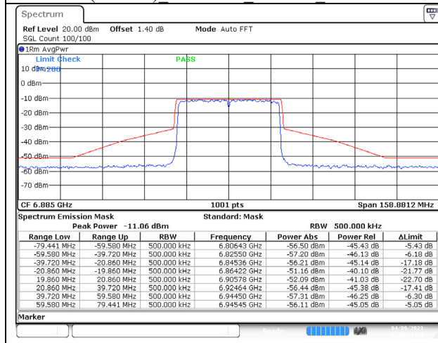
802.11ax (40MHz) 6885MHz Chain A NSS-4
