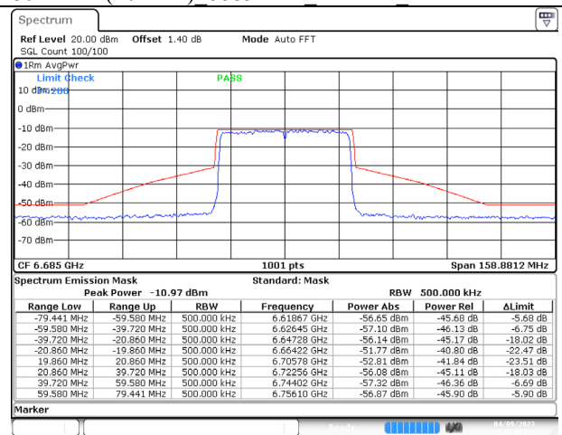
802.11ax (40MHz) 6685MHz Chain D NSS-4
