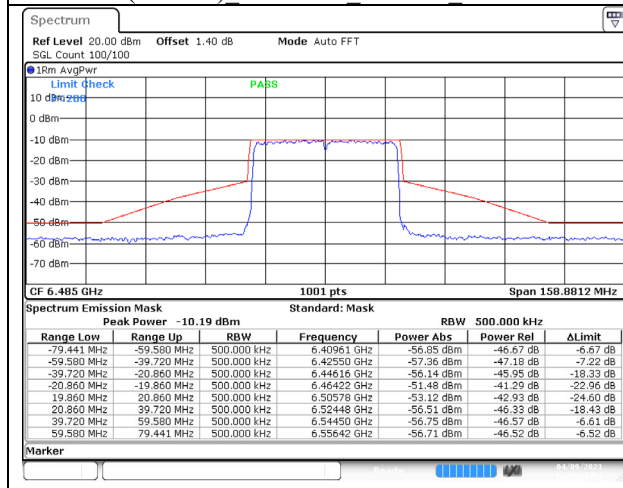
802.11ax (40MHz) 6485MHz Chain C NSS-4
