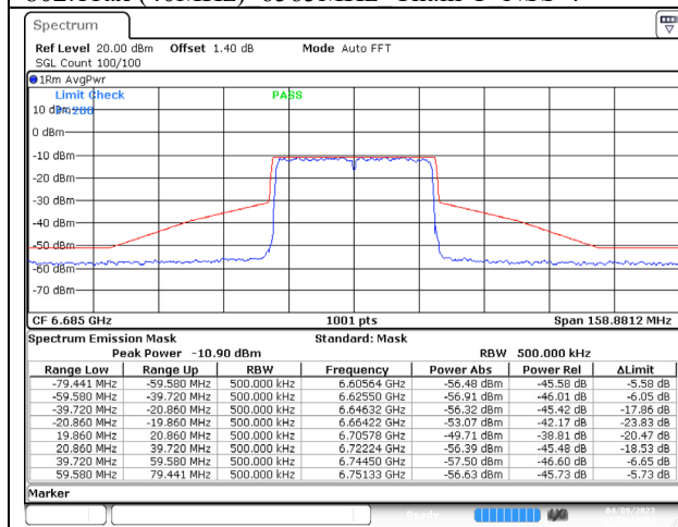
802.11ax (40MHz) 6685MHz Chain A NSS-4
