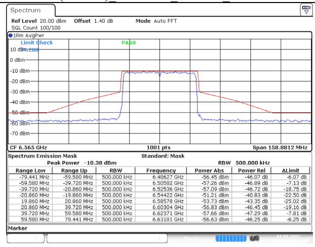
802.11ax (40MHz) 6565MHz Chain B NSS-4
