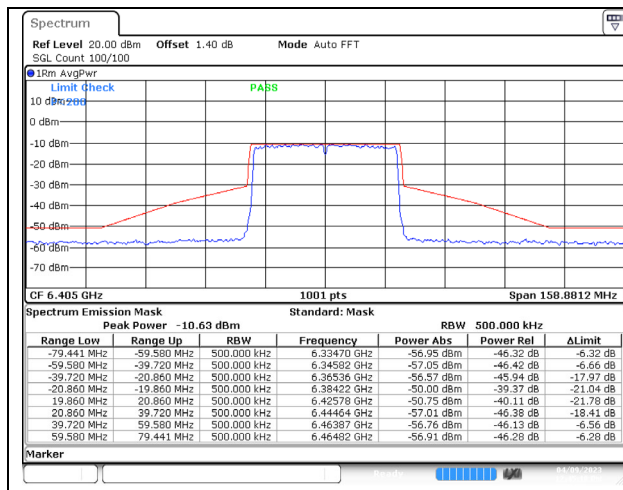
802.11ax (40MHz) 6405MHz Chain A NSS-4
