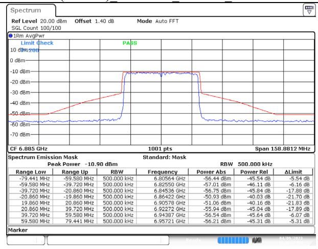
802.11ax (40MHz) 6885MHz Chain B NSS-4
