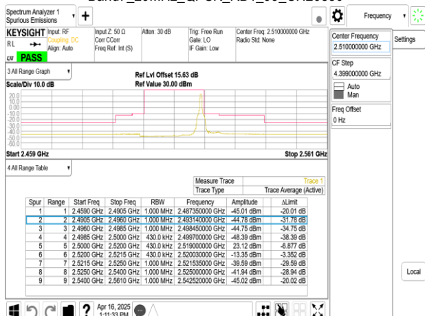
Band7_20MHz_QPSK_RB1_99_CH20850
