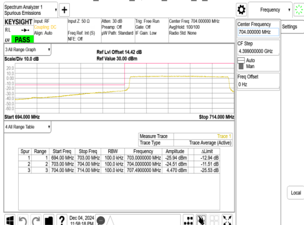
Band17_10MHz_QPSK_RB1_49_CH23800
