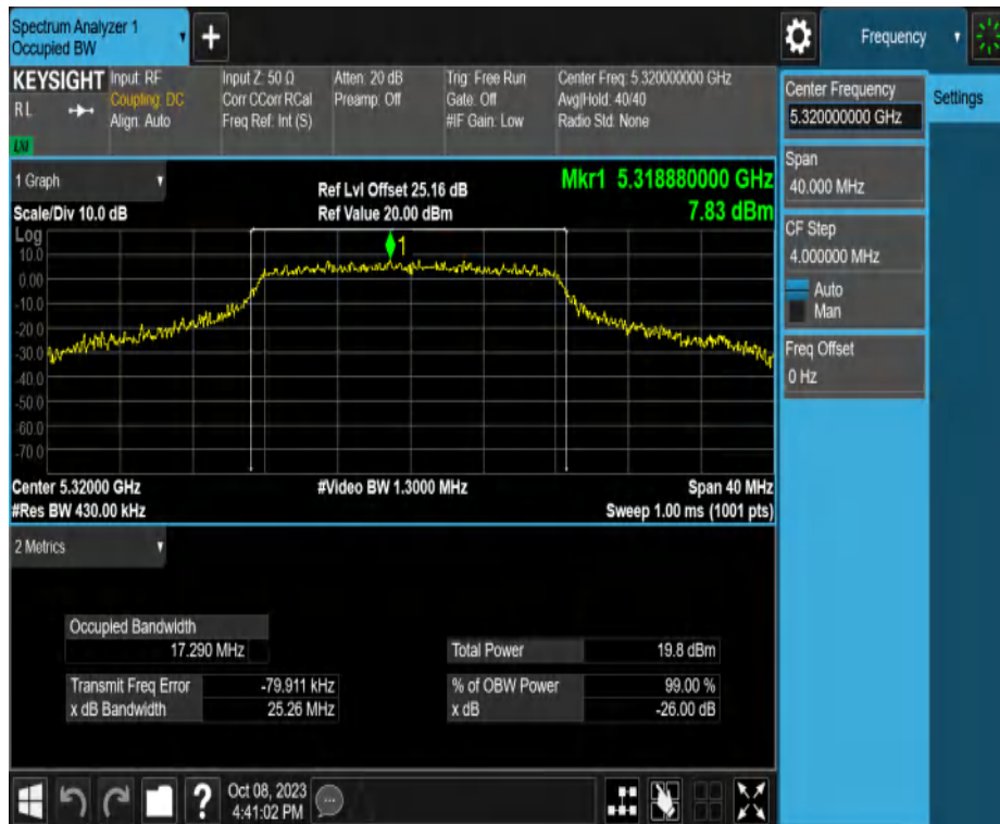
11A-CDD_Ant2_5320
