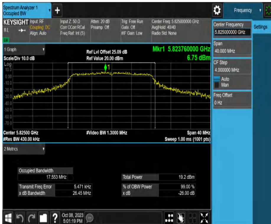
11A-CDD_Ant2_5825
