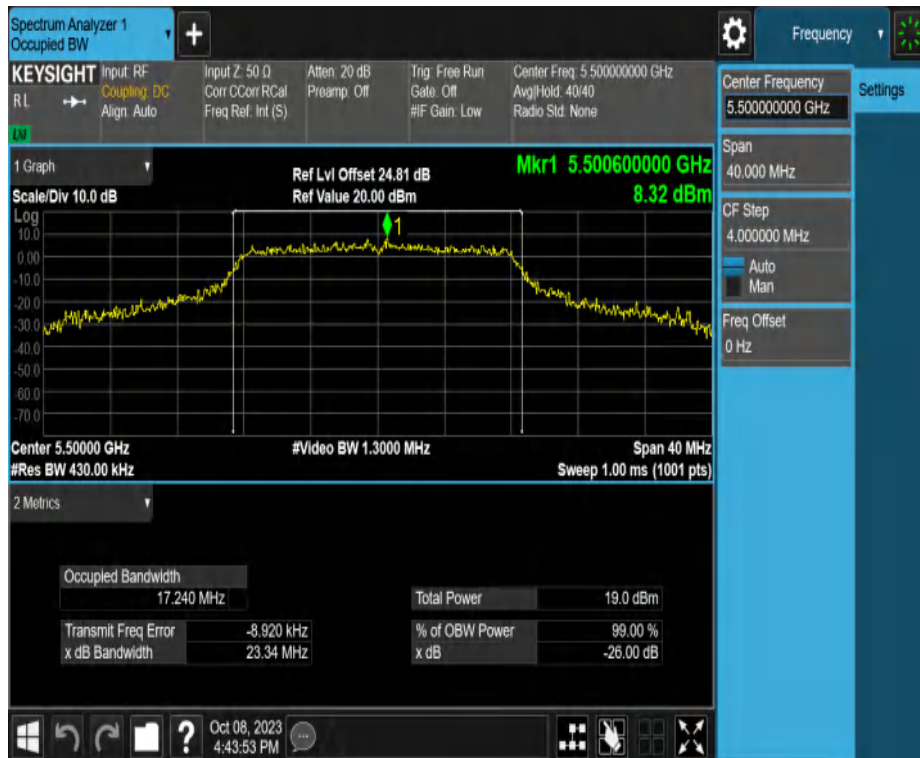
11A-CDD_Ant2_5500
