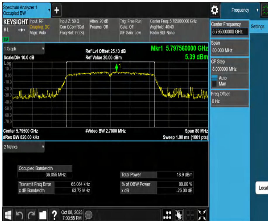
11N40MIMO_Ant2_5795
