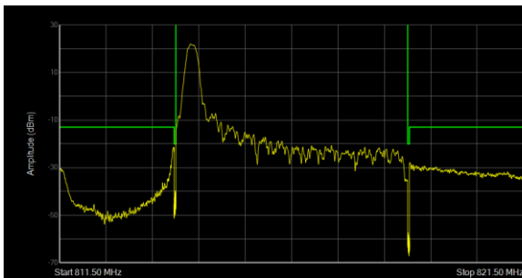
LTE Band 26 QPSK 5MHz CH-Low 1RB
