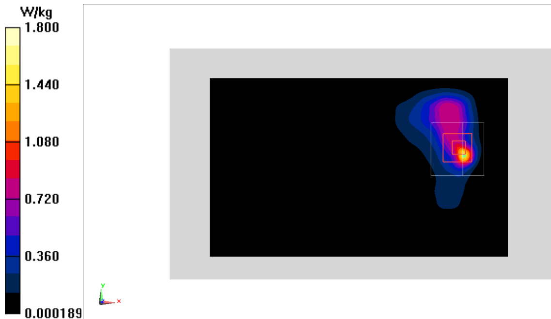
Fig.14 LTE Band38
