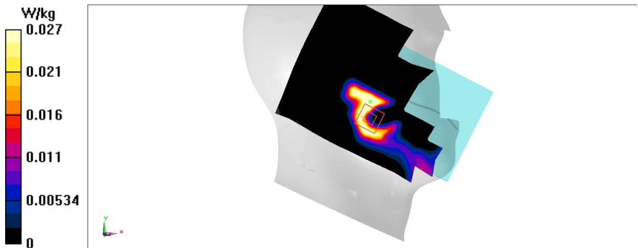
Fig.13 LTE Band38
