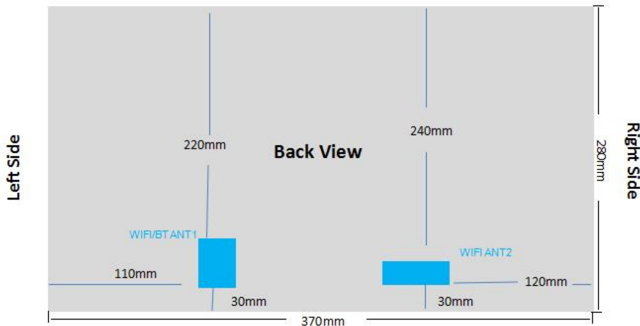
Bottom Side
