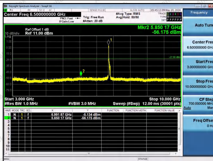
11AX80SISO-Ant1-7025-242Tone-RU61-3000~10000-PASS
