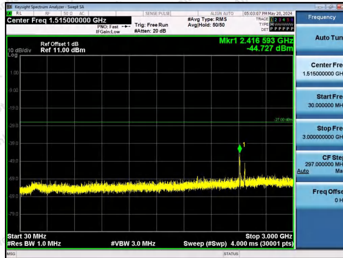
11AX80SISO-Ant1-6945-26Tone-RU0-30~3000-PASS
