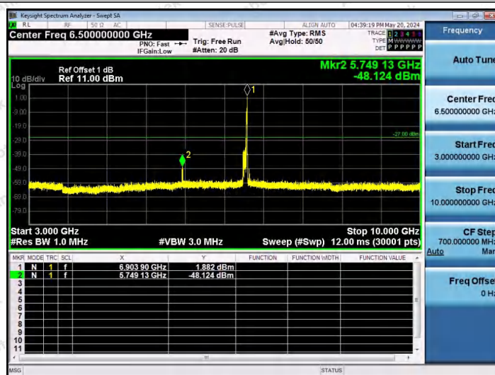
11AX80SISO-Ant1-6865-26Tone-RU36-3000~10000-PASS
