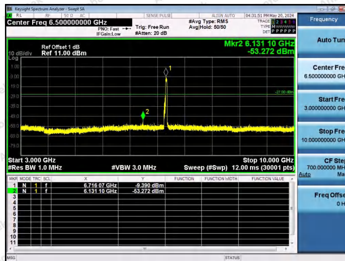
11AX80SISO-Ant1-6705-484Tone-RU66-3000~10000-PASS
