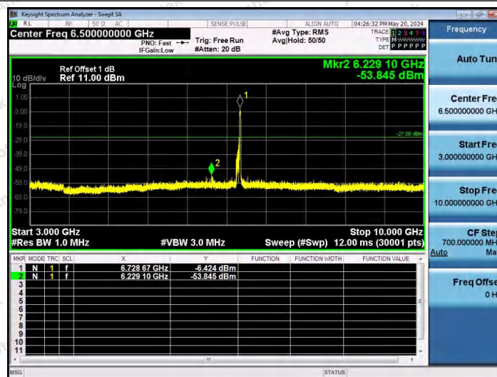
11AX80SISO-Ant1-6705-242Tone-RU64-3000~10000-PASS
