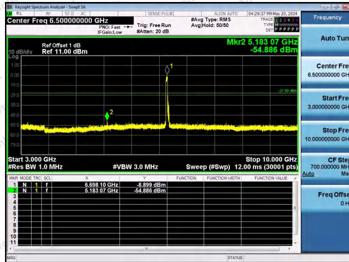
11AX80SISO-Ant1-6705-484Tone-RU65-3000~10000-PASS
