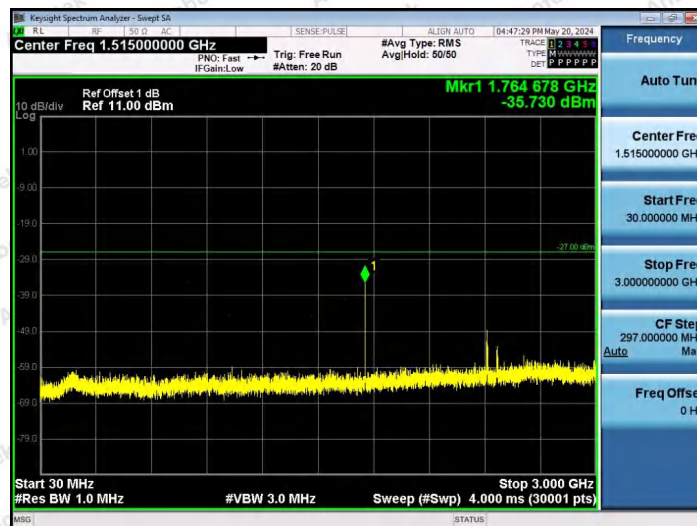
11AX80SISO-Ant1-6865-106Tone-RU53-30~3000-PASS
