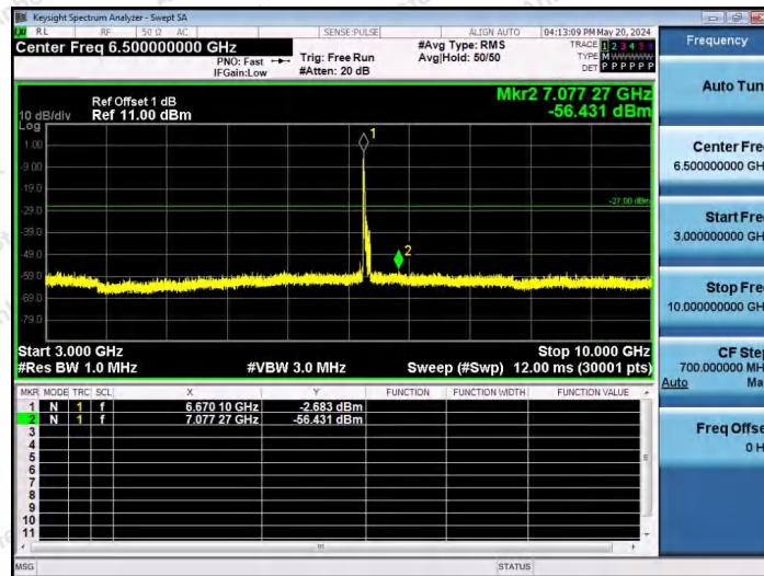
11AX80SISO-Ant1-6705-52Tone-RU37-3000~10000-PASS
