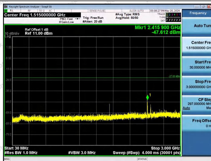
11AX80SISO-Ant1-6945-52Tone-RU37-30~3000-PASS
