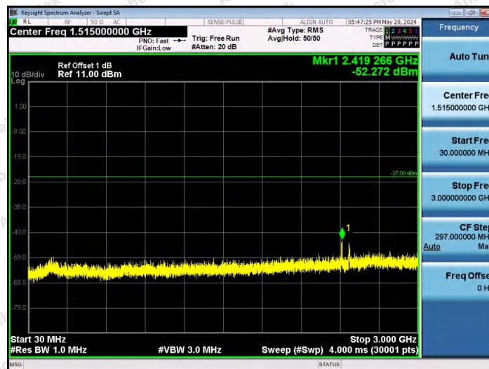
11AX80SISO-Ant1-7025-242Tone-RU64-30~3000-PASS
