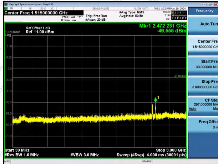
11AX80SISO-Ant1-6945-52Tone-RU52-30~3000-PASS
