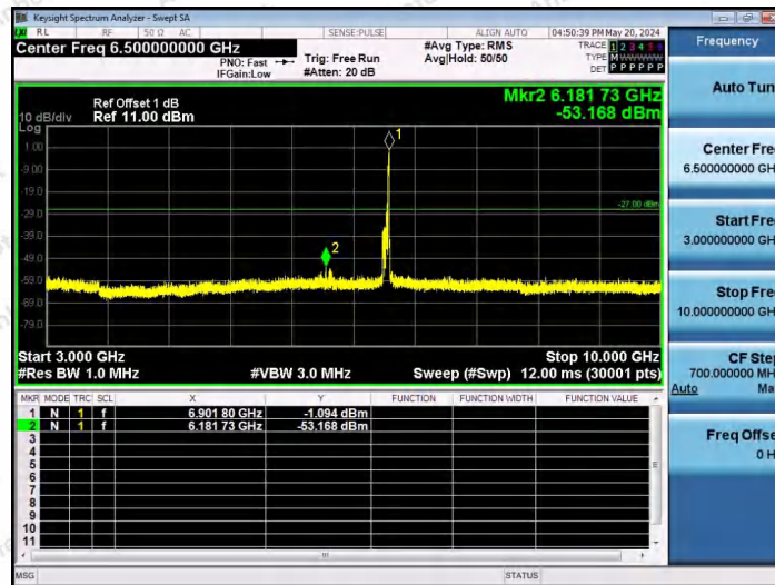
11AX80SISO-Ant1-6865-106Tone-RU60-3000~10000-PASS
