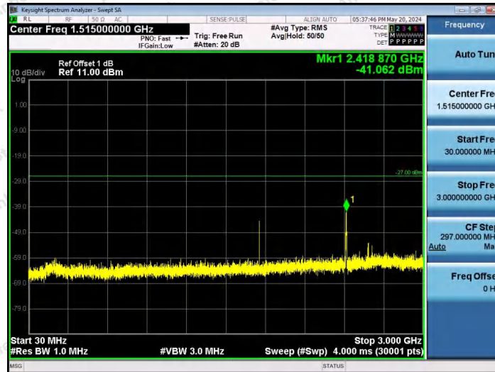
11AX80SISO-Ant1-7025-52Tone-RU52-30~3000-PASS
