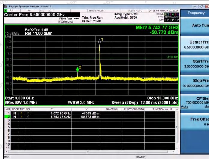
11AX80SISO-Ant1-6705-106Tone-RU53-3000~10000-PASS
