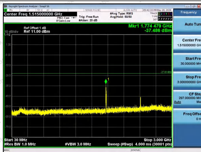
11AX80SISO-Ant1-7025-106Tone-RU60-30~3000-PASS
