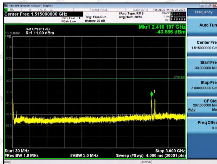
11AX80SISO-Ant1-6945-242Tone-RU64-30~3000-PASS
