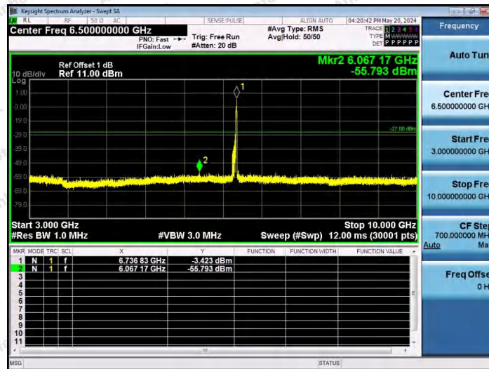
11AX80SISO-Ant1-6705-106Tone-RU60-3000~10000-PASS
