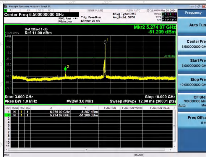
11AX80SISO-Ant1-6945-242Tone-RU64-3000~10000-PASS
