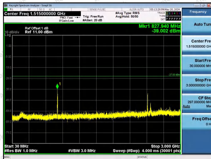
11AX80SISO-Ant1-6945-106Tone-RU53-30~3000-PASS
