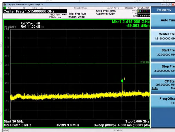
11AX80SISO-Ant1-6865-242Tone-RU64-30~3000-PASS
