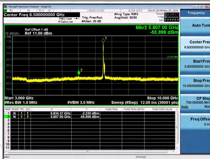
11AX80SISO-Ant1-6865-106Tone-RU53-3000~10000-PASS
