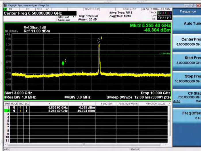
11AX80SISO-Ant1-6865-484Tone-RU65-3000~10000-PASS
