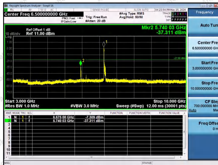
11AX80SISO-Ant1-6705-242Tone-RU61-3000~10000-PASS
