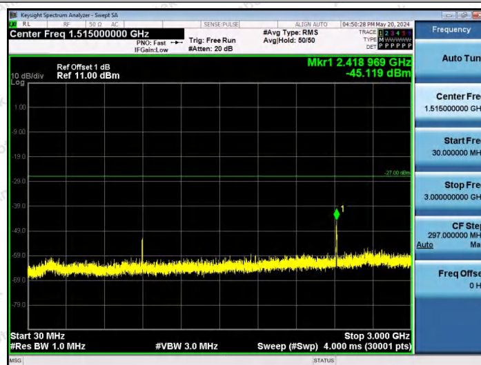
11AX80SISO-Ant1-6865-106Tone-RU60-30~3000-PASS
