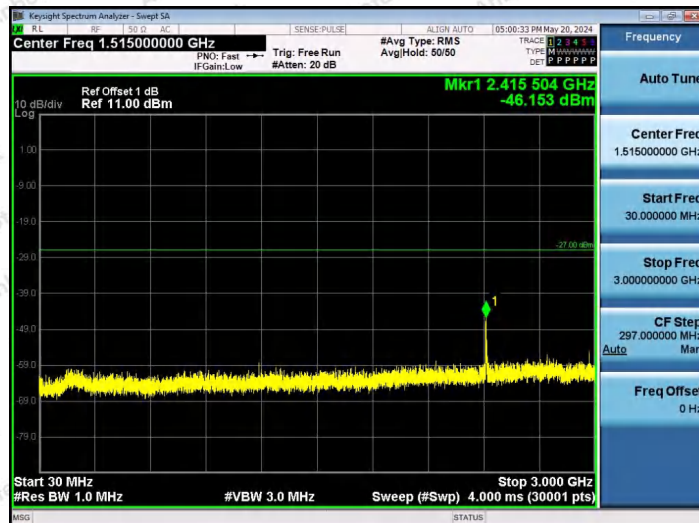
11AX80SISO-Ant1-6865-484Tone-RU66-30~3000-PASS
