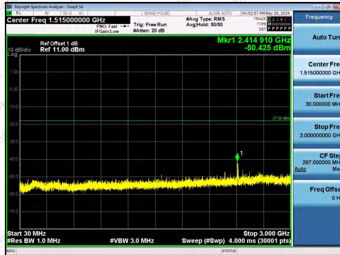
11AX80SISO-Ant1-6865-242Tone-RU61-30~3000-PASS
