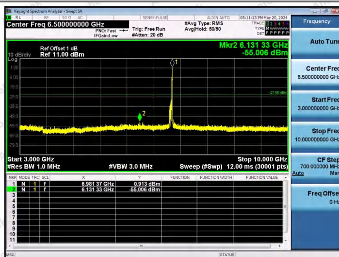
11AX80SISO-Ant1-6945-52Tone-RU52-3000~10000-PASS
