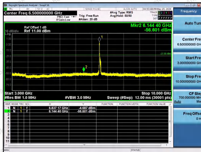
11AX80SISO-Ant1-6865-242Tone-RU61-3000~10000-PASS
