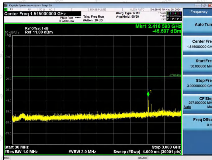
11AX80SISO-Ant1-6865-26Tone-RU36-30~3000-PASS
