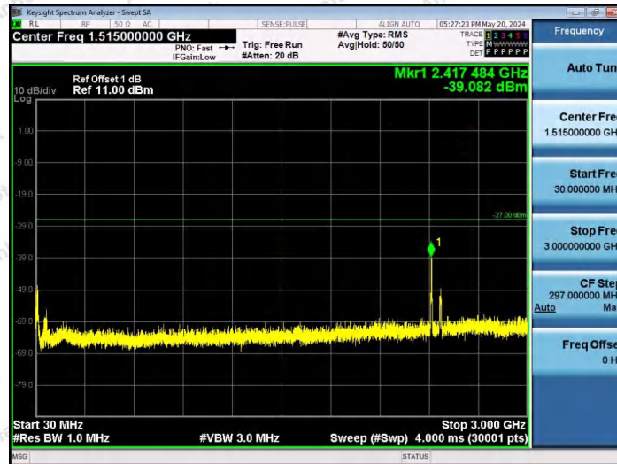
11AX80SISO-Ant1-6945-484Tone-RU66-30~3000-PASS
