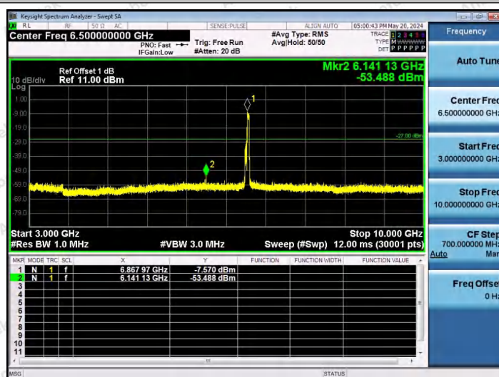
11AX80SISO-Ant1-6865-484Tone-RU66-3000~10000-PASS
