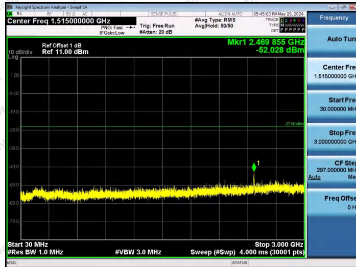
11AX80SISO-Ant1-7025-242Tone-RU61-30~3000-PASS
