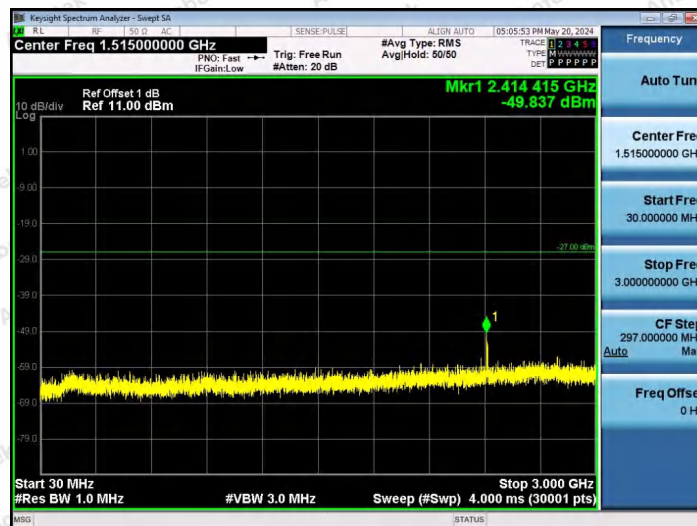
11AX80SISO-Ant1-6945-26Tone-RU36-30~3000-PASS
