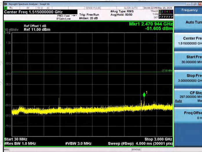
11AX80SISO-Ant1-6865-52Tone-RU52-30~3000-PASS
