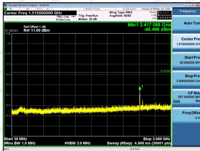
11AX80SISO-Ant1-7025-106Tone-RU53-30~3000-PASS
