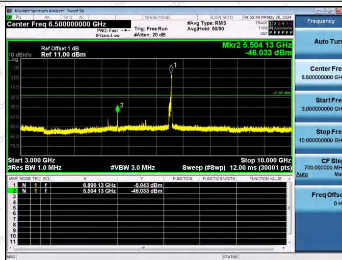
11AX80SISO-Ant1-6865-242Tone-RU64-3000~10000-PASS
