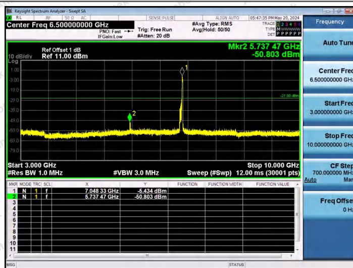
11AX80SISO-Ant1-7025-242Tone-RU64-3000~10000-PASS
