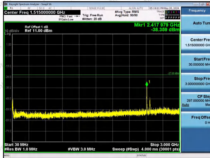
11AX80SISO-Ant1-6945-242Tone-RU61-30~3000-PASS
