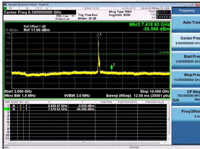
11AX80SISO-Ant1-6865-52Tone-RU37-3000~10000-PASS
