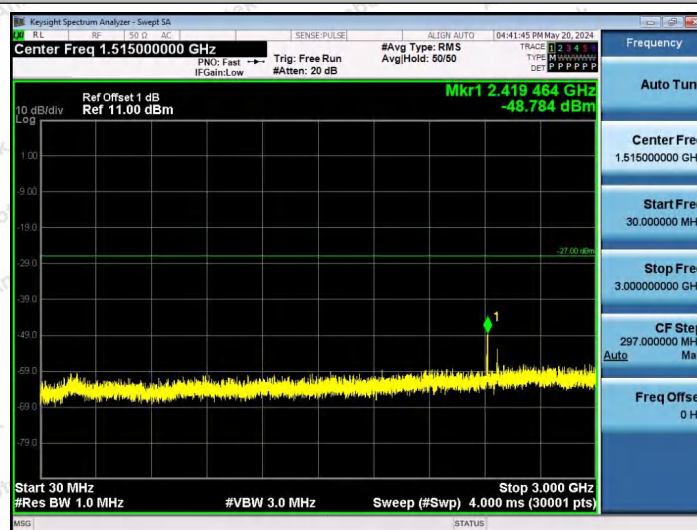
11AX80SISO-Ant1-6865-52Tone-RU37-30~3000-PASS
