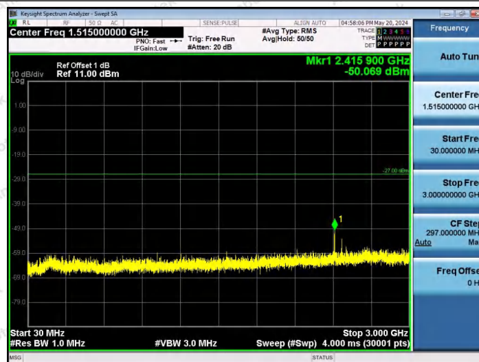
11AX80SISO-Ant1-6865-484Tone-RU65-30~3000-PASS
