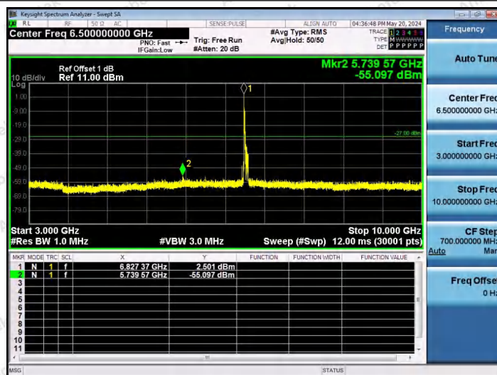
11AX80SISO-Ant1-6865-26Tone-RU0-3000~10000-PASS
