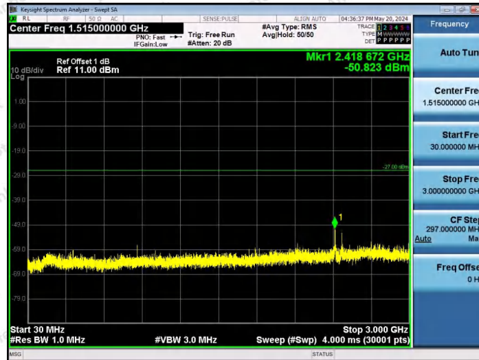
11AX80SISO-Ant1-6865-26Tone-RU0-30~3000-PASS
