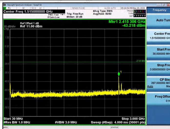
11AX80SISO-Ant1-6945-484Tone-RU65-30~3000-PASS
