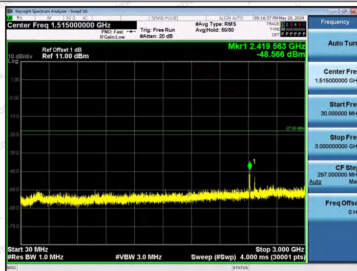
11AX80SISO-Ant1-6945-106Tone-RU60-30~3000-PASS
