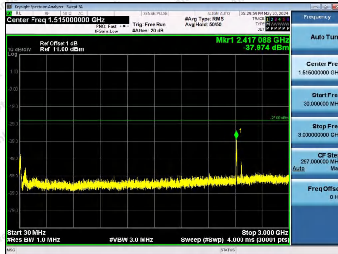
11AX80SISO-Ant1-7025-26Tone-RU0-30~3000-PASS
