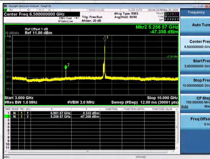
11AX80SISO-Ant1-6865-52Tone-RU52-3000~10000-PASS
