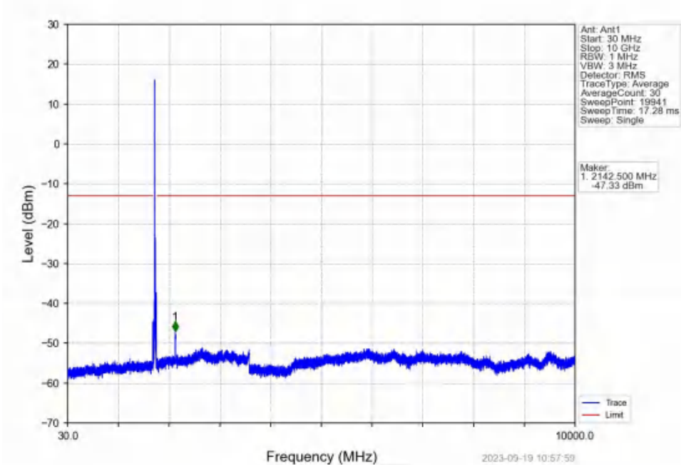
Band4_20MHz_QPSK_HCH_1745MHz_RB_1_0_NTNV
