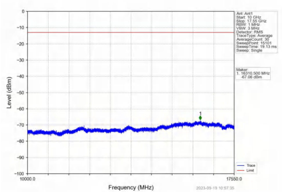
Band4_20MHz_QPSK_MCH_1732.5MHz_RB_1_0_NTNV
