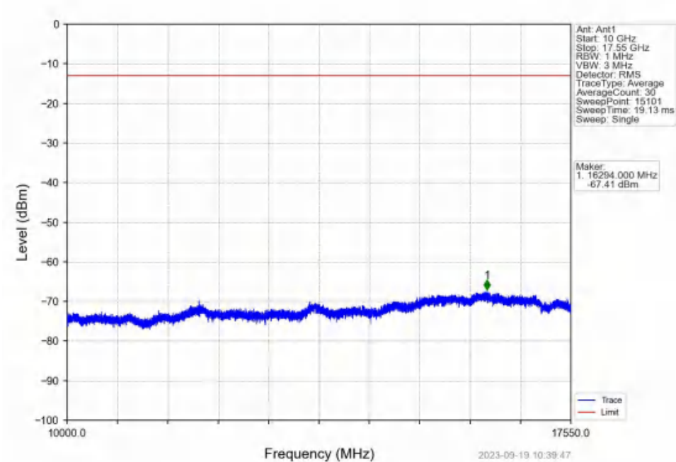
Band4_15MHz_QPSK_LCH_1717.5MHz_RB_1_0_NTNV
