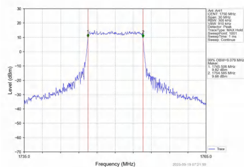
Band4_10MHz_QPSK_HCH_1750MHz_RB_50_0_NTNV
