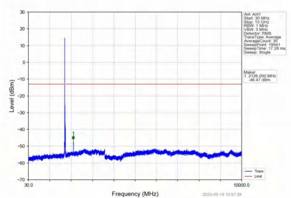
Band4_20MHz_QPSK_MCH_1732.5MHz_RB_1_0_NTNV
