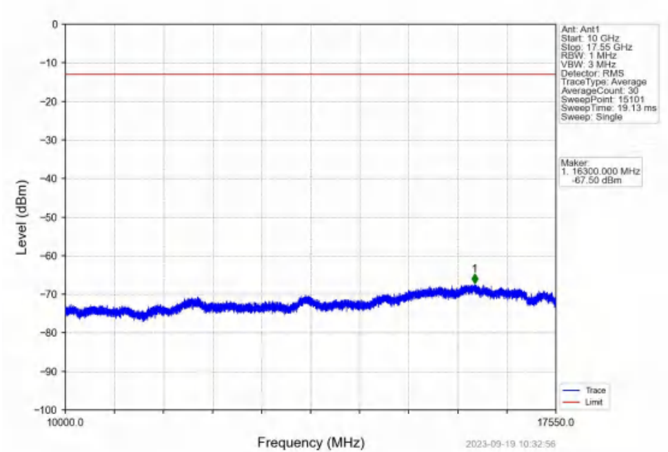
Band4_10MHz_QPSK_HCH_1750MHz_RB_1_0_NTNV
