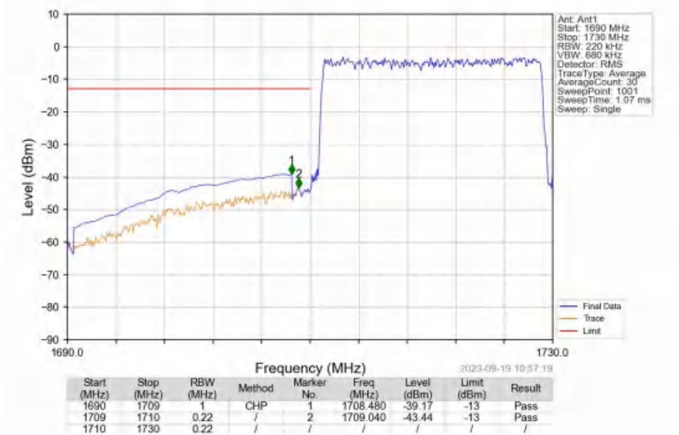
Band4_20MHz_16QAM_LCH_1720MHz_RB_100_0_NTNV
