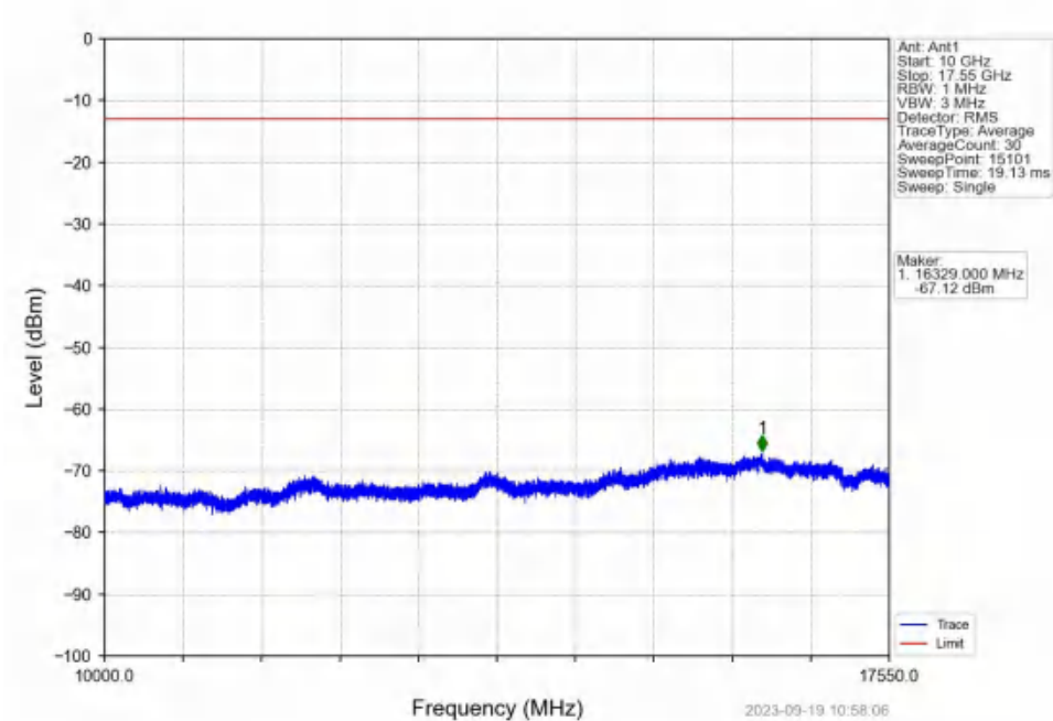
Band4_20MHz_QPSK_HCH_1745MHz_RB_1_0_NTNV
