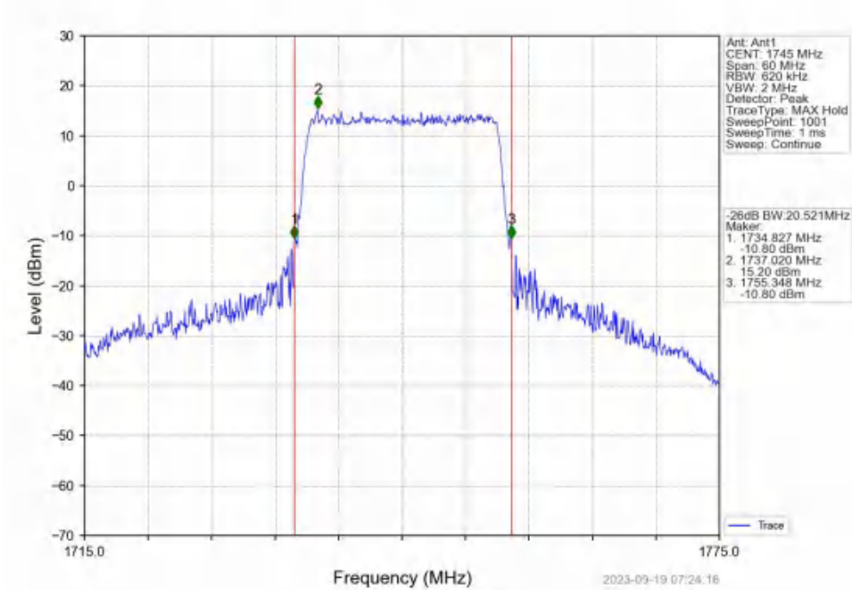
Band4_20MHz_QPSK_HCH_1745MHz_RB_100_0_NTNV
