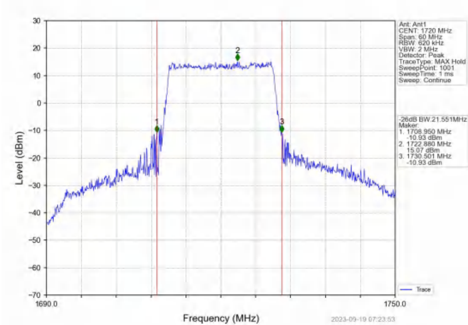
Band4_20MHz_16QAM_LCH_1720MHz_RB_100_0_NTNV
