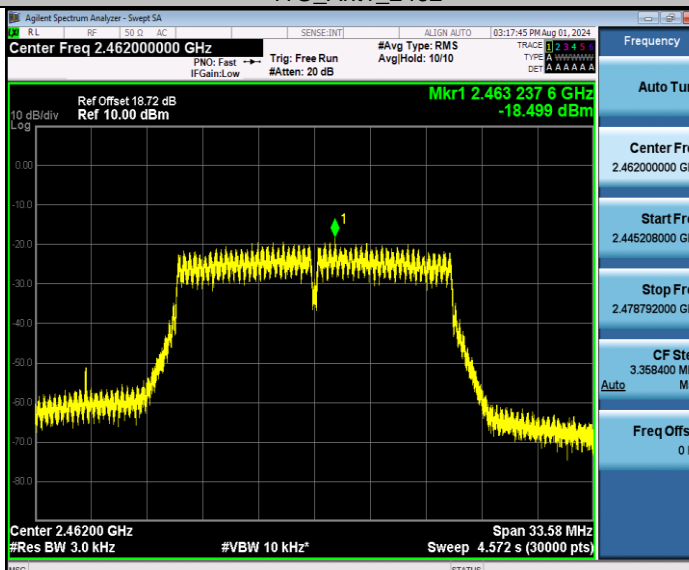
11G_Ant1_2462
