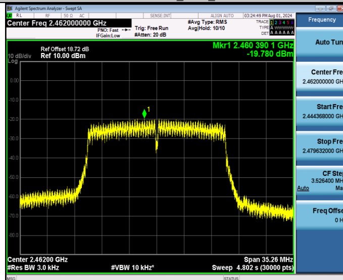
11N20SISO_Ant1_2462
