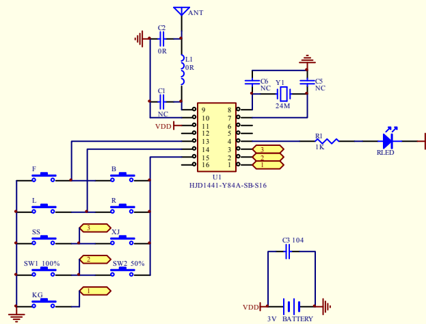
DLXH-Z6750TX-2.4G原理图
