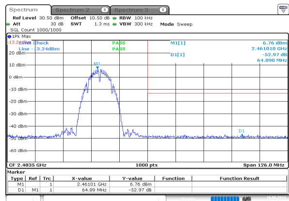
b_2462MHz_Chain 0
