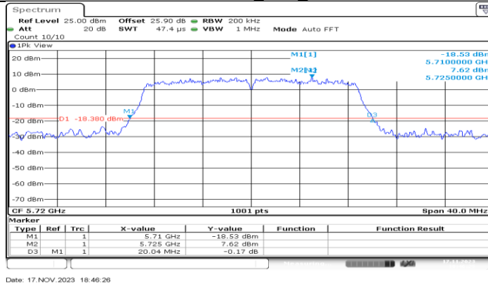
11N20MIMO Ant1 5720
