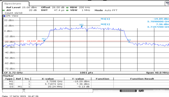
11N20MIMO Ant2 5720
