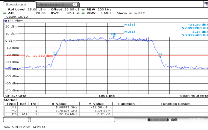
11N20MIMO Ant1 5700
