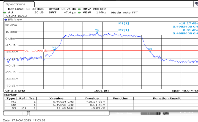
11A-CDD_Ant1_5500
