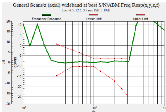
Fig. 7.6 LTE Band 2
