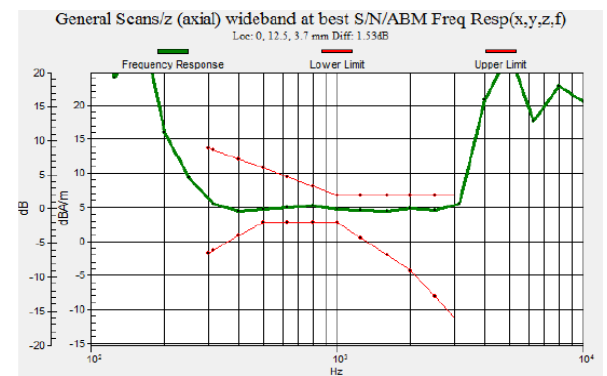
Fig. 7.12 LTE Band 4
