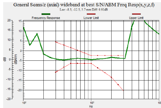
Fig. 7.15 LTE Band 4
