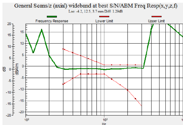
Fig. 7.11 LTE Band 4
