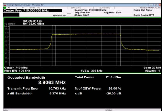
FDD17_MidRange_10_710_Q16
