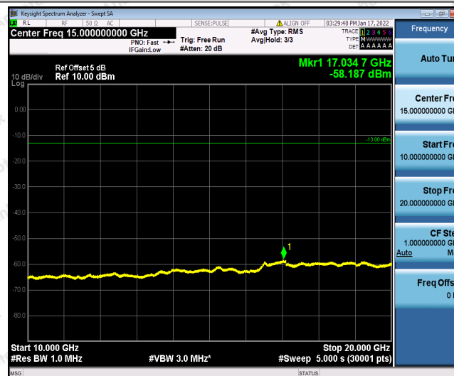
Band2-9538-1-10000~20000MHz
