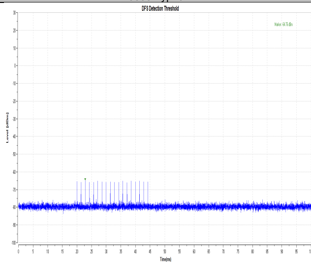
11AC80SISO-5290-Type0-PASS
