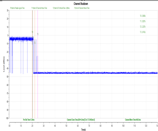
11AC80SISO-5290-Type0-PASS
