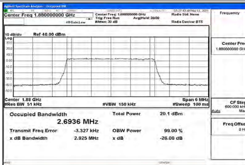
Band2-3MHz-QPSK-19185-15RB#0-2.6924
