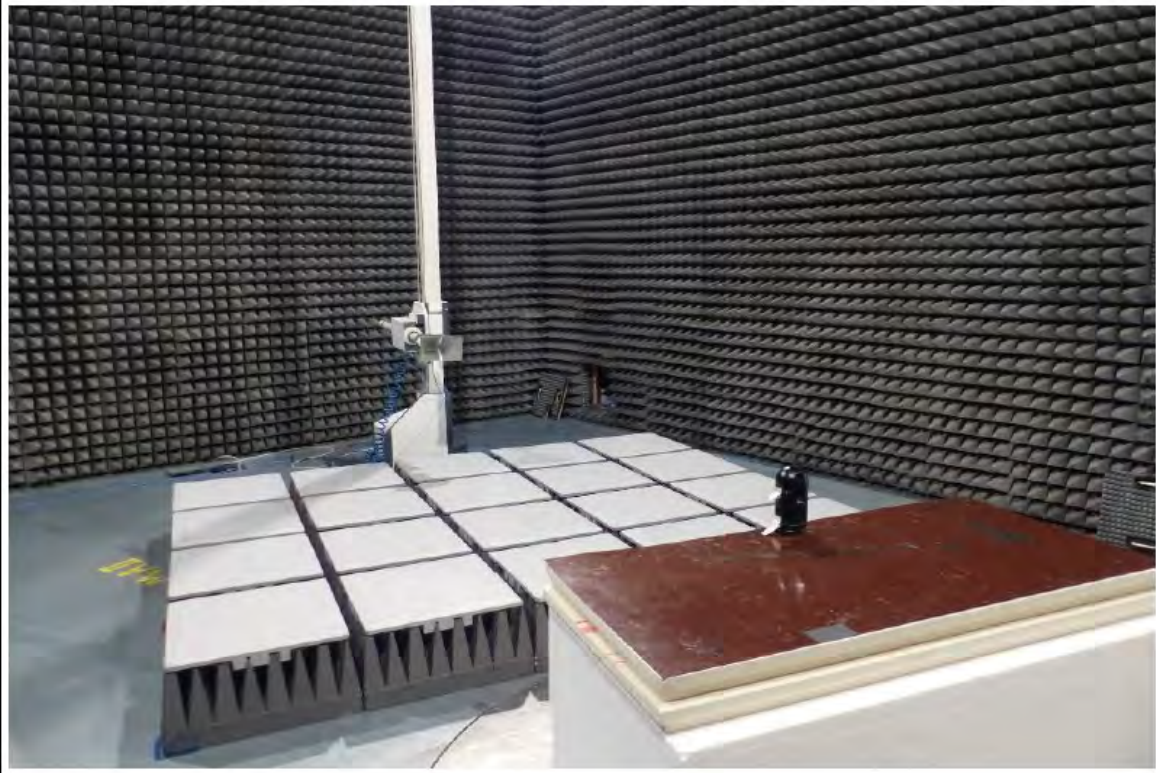
Test setup EUT Configuration I: 1000-17000MHz
