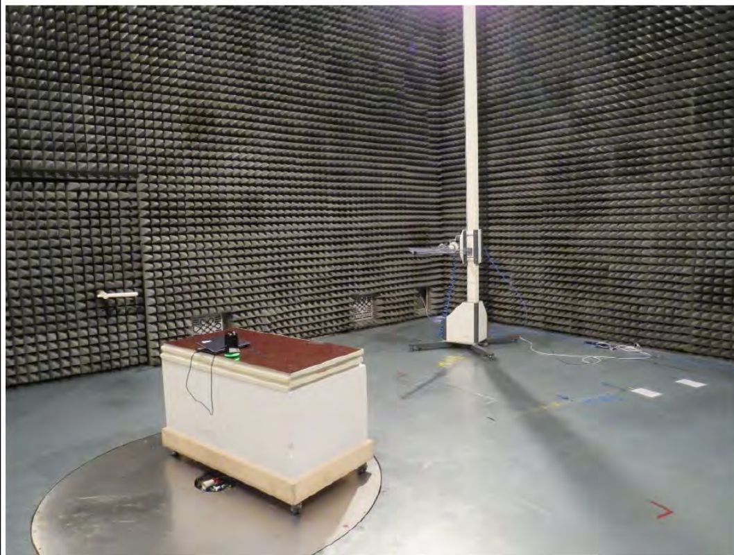
Setup 200 - 1000MHz
