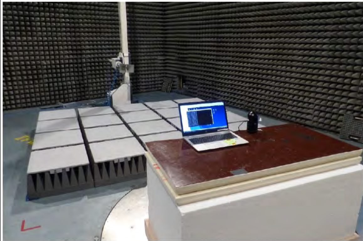
Test setup EUT Configuration II: 1000-17000MHz
