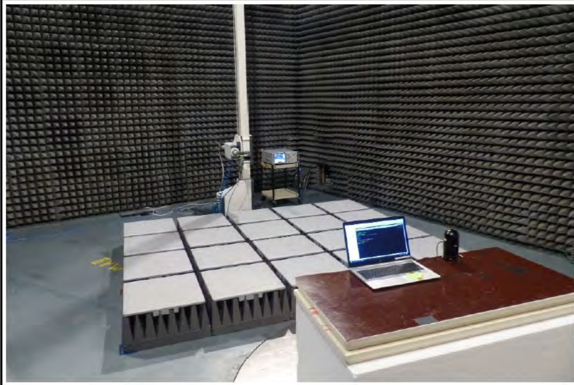
Test setup EUT Configuration II: 26500-30000MHz
