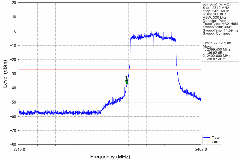
802.11ax(HEW40)_LCH_2422MHz_SU_/_Ant0 (MIMO)_NTNV
