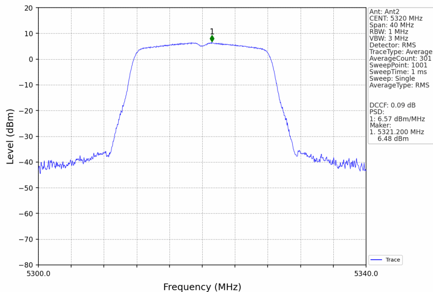
802.11a_HCH_5320MHz_Ant2_NTNV
