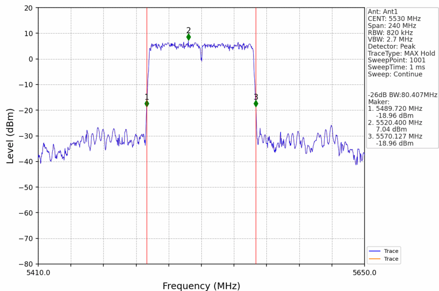
802.11ax(HEW80)_LCH_5530MHz_RU996_Left_Ant1_NTNV
