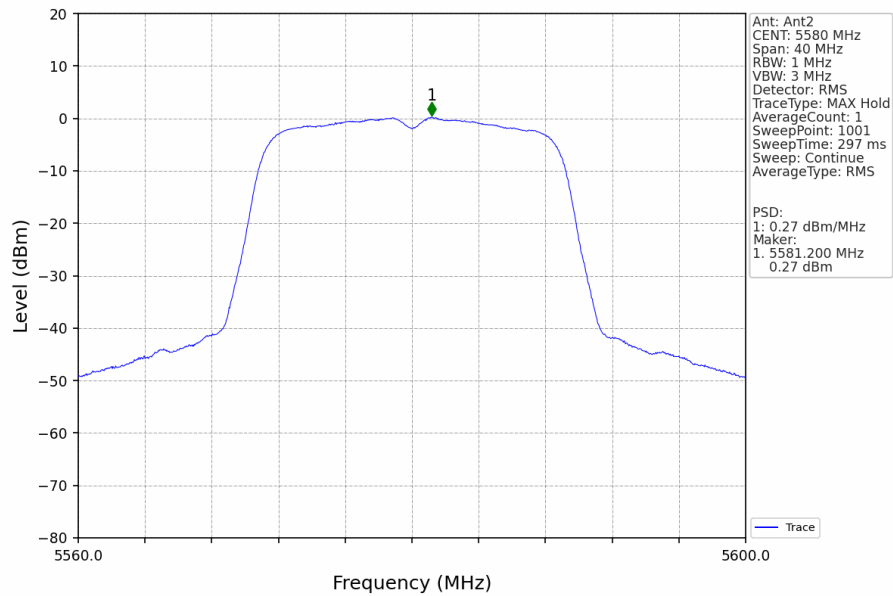
802.11n(HT20)_MCH_5580MHz_MIMO_NTNV
