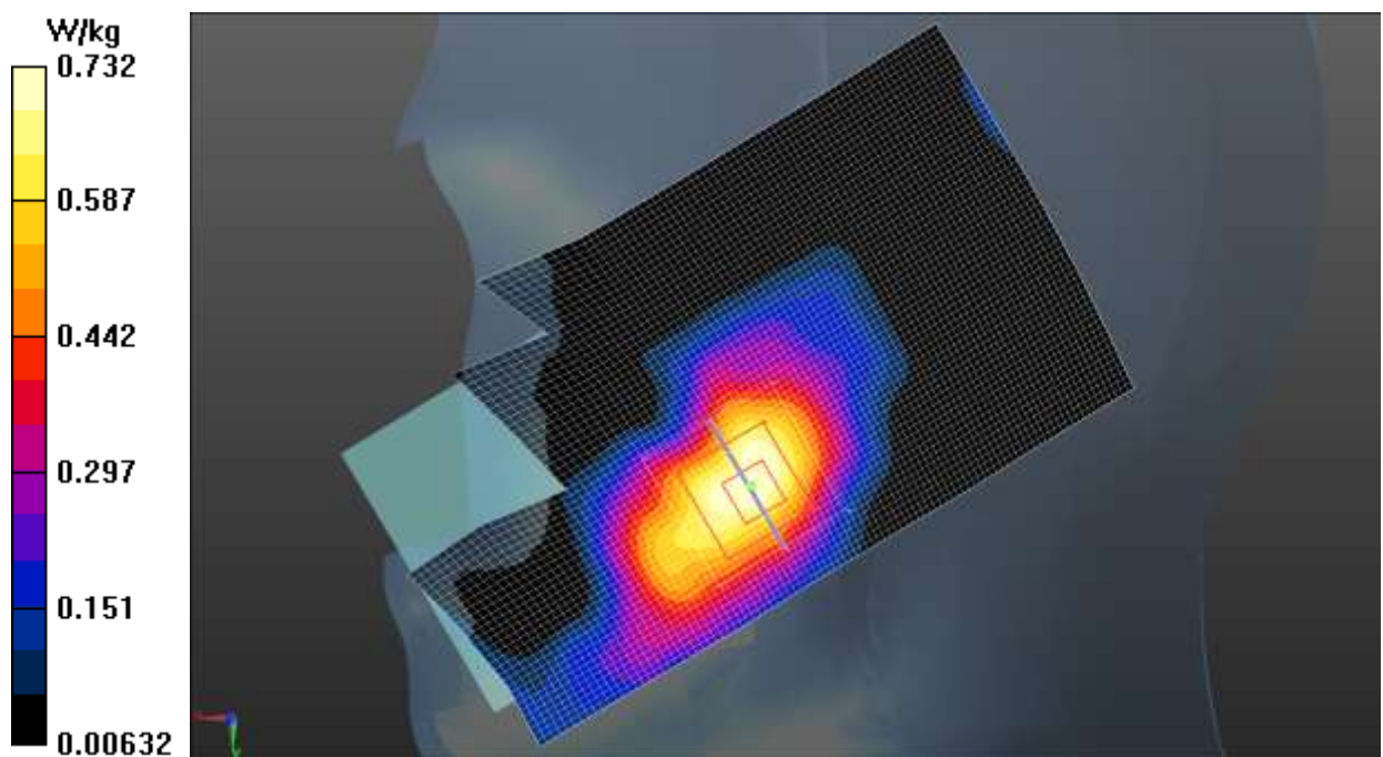
Fig.7 CDMA BC1
