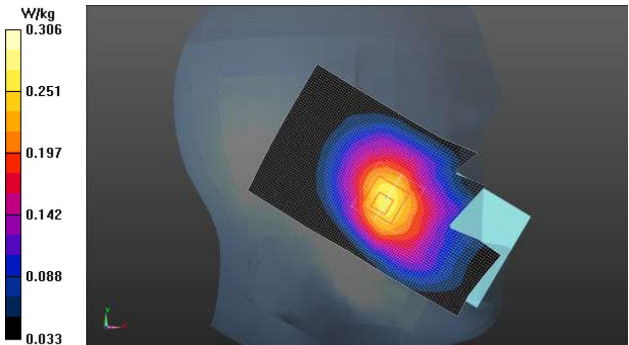
Fig.9 CDMA BC10
