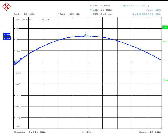
GFSK_ANT1_2441
