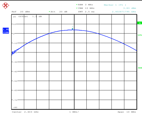
GFSK_ANT1_2403
