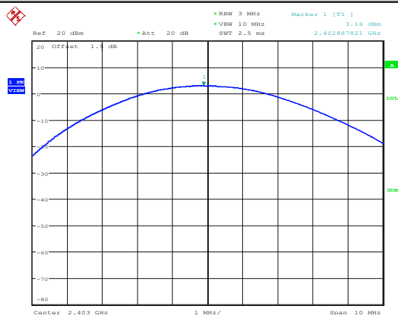
GFSK_ANT2_2403
