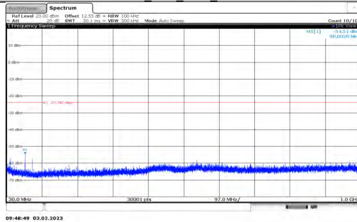
11N20SISO_Ant1_2457_30~1000
