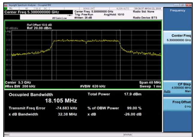
U-NII-2a 26dB Bandwidth-802.11ac(20MHz z) ,5300MHz
