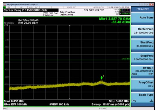
U-NII-2a ,Plot 2,30MHz~5000MHz-802.11 n(40MHz),5310MHz
