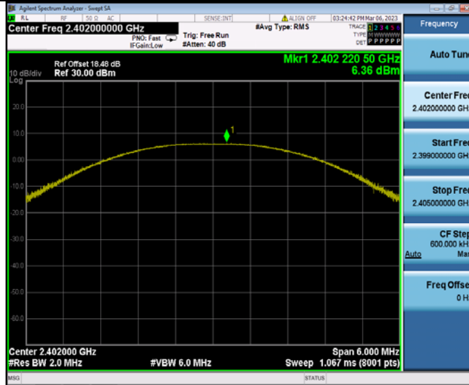
SRD2.4G Ant2_2402
