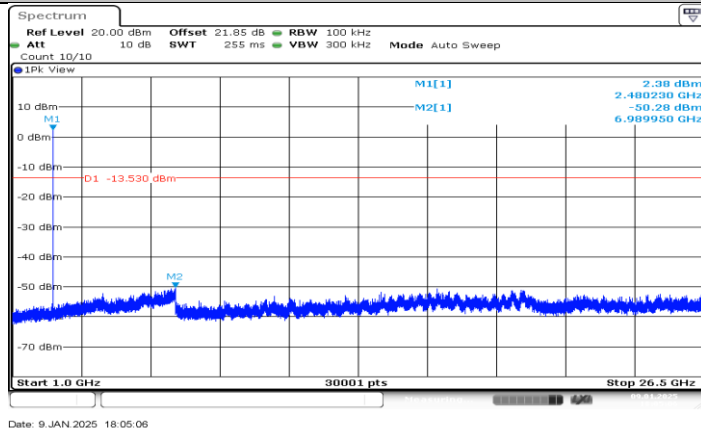
BLE_2M_Ant BT_2480_1000~26500
