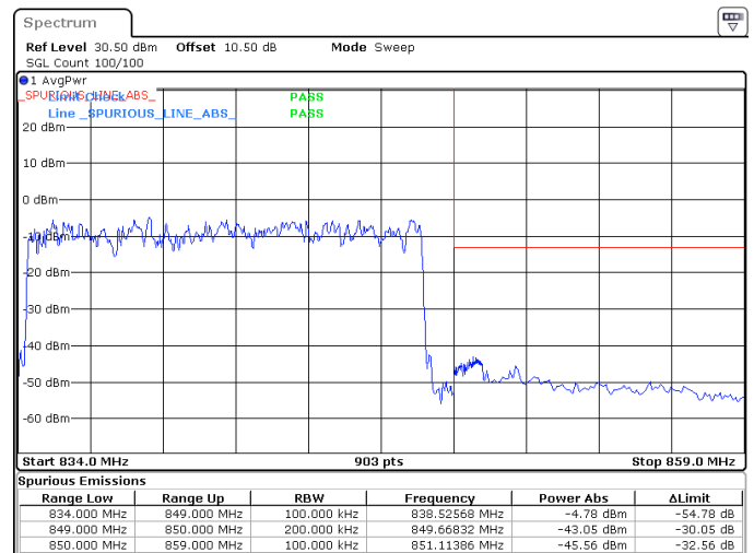
15MHz_15kHz_841.5MHz_DFT-s-OFDM QPSK_RB75@0 -43.05 dBm
