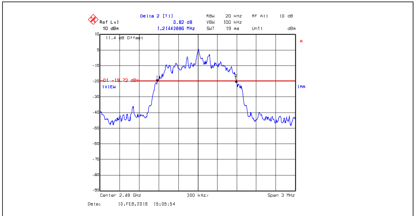
Plot 5.3.4.1.12. 20 dB Bandwidth, \pi/4 -DQPSK, 2DH1, CH 78, 2480 MHz
