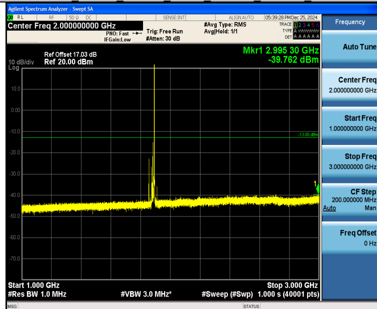
Band25 20MHz 16QAM 26365 1RB#99 1000~3000 1000~3000
