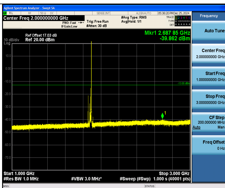
Band25 20MHz QPSK 26365 1RB#99 1000~3000 1000~3000
