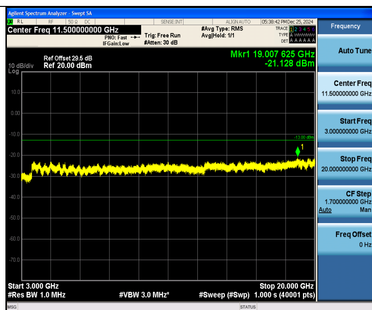
Band25 20MHz QPSK 26365 1RB#99 3000~20000 3000~20000
