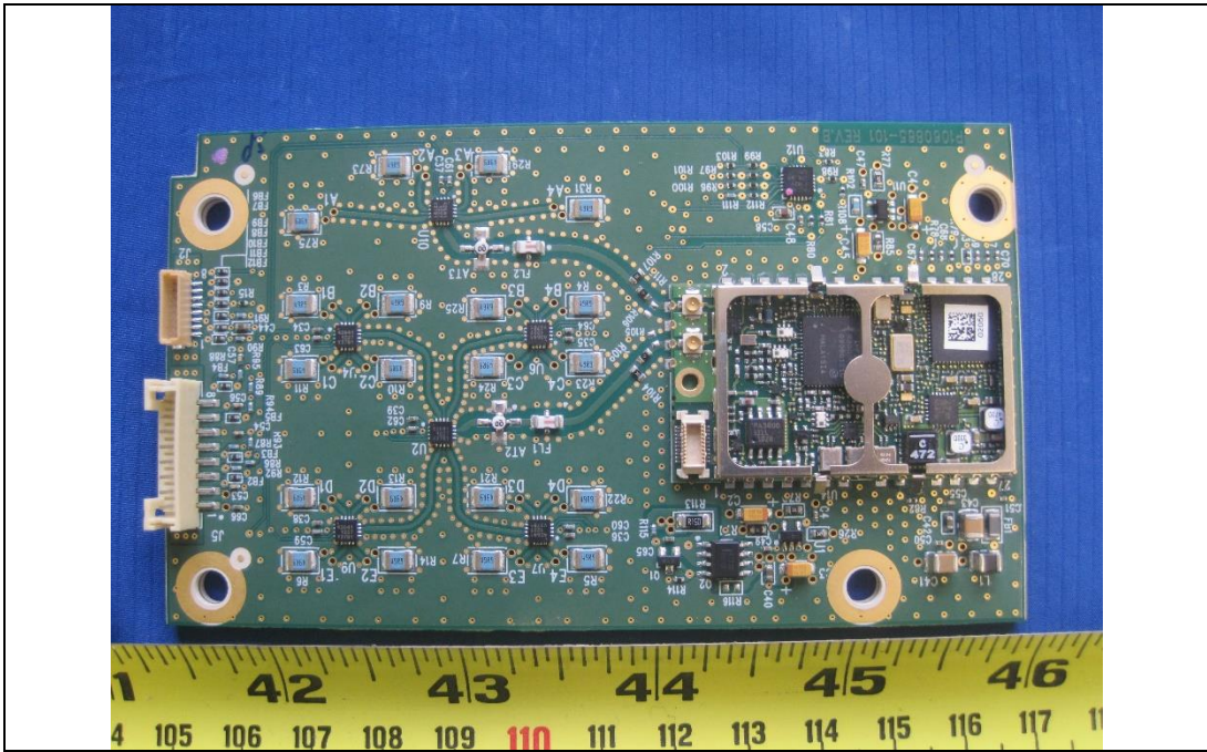
RFID module Top View
