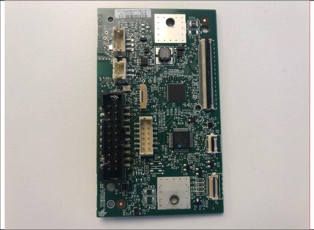
Radio Module PCBA back
