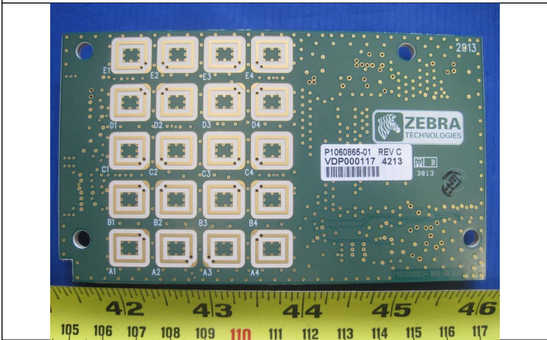
RFID module Bottom View
