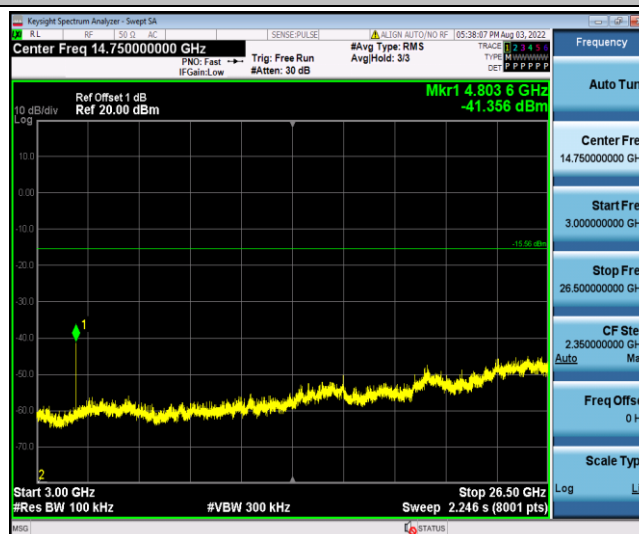
BLE_BT5.0_Ant2_2402_3000~26500
