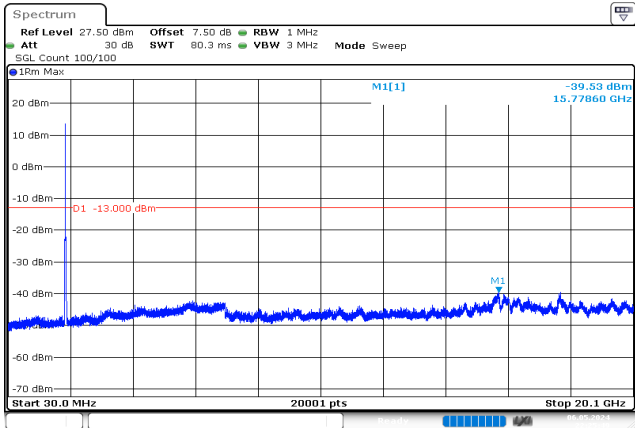
20MHz_Low_QPSK_100@0 -39.53 dBm
