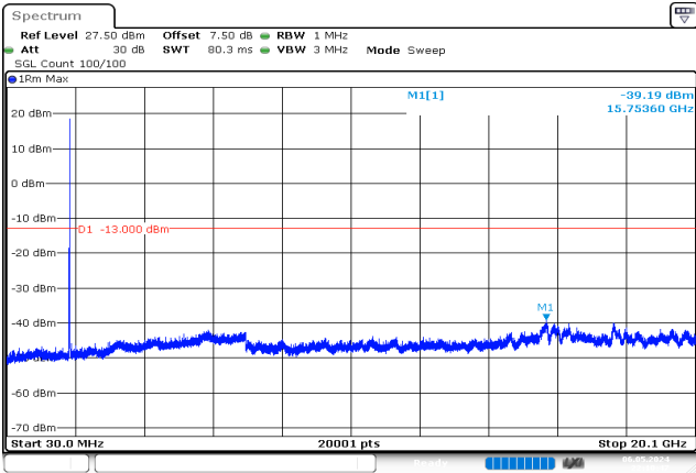
5MHz_Low_QPSK_25@0 -39.19 dBm
