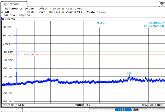
5MHz_Middle_QPSK_25@0 -39.20 dBm
