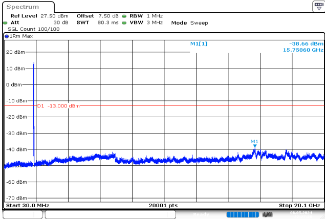
20MHz_Middle_QPSK_100@0 -38.66 dBm
