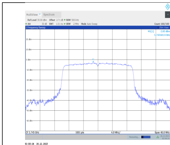
11ax20MIMO-Ant3-5745-PASS
