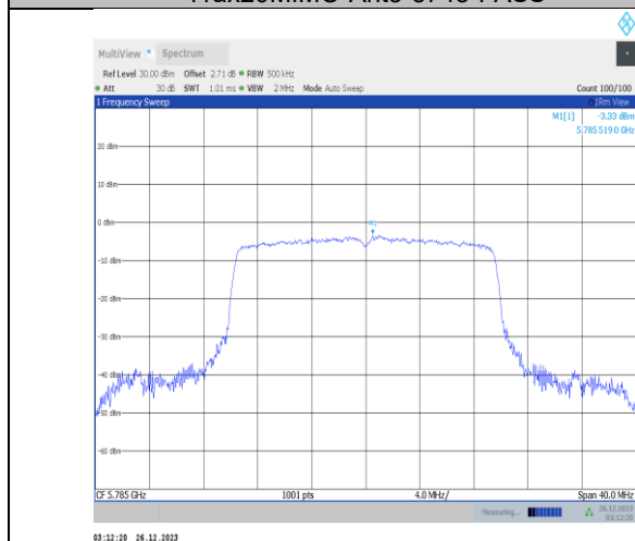
11ax20MIMO-Ant1-5785-PASS
