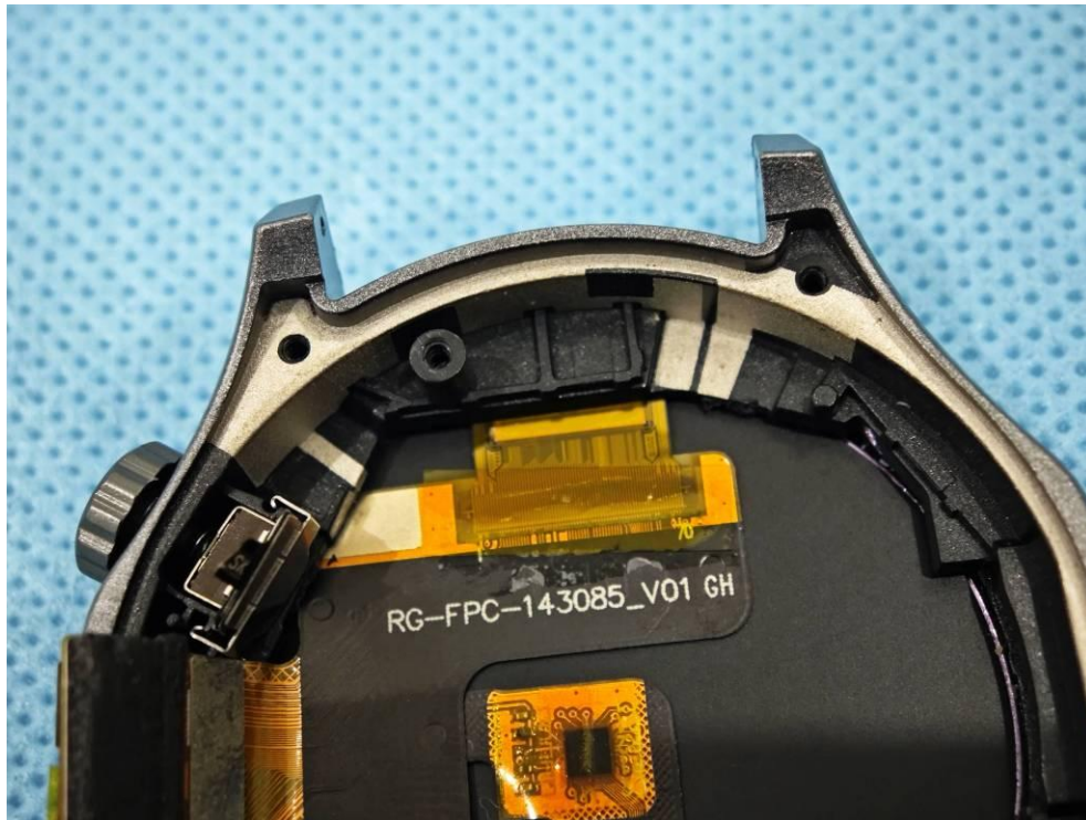
GSM&LTE ANT
